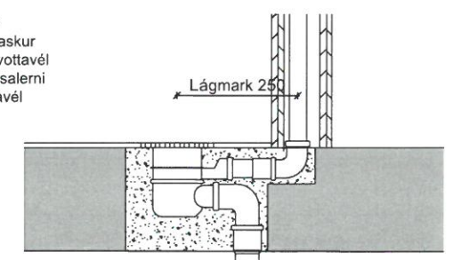
GÓLFNIÐURFALL MEÐ GEGNURENNSLI, MKV.:1:10
