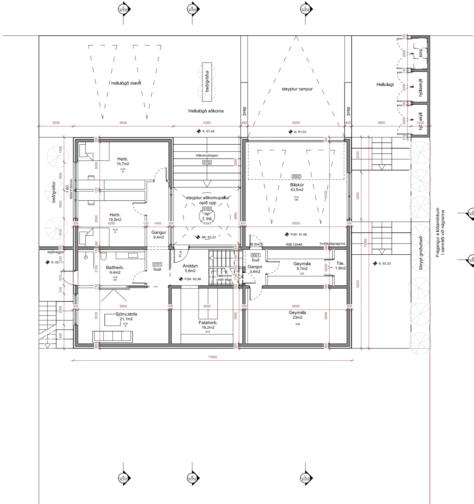
Grunnmynd neðri hæða mkv: 1:100
