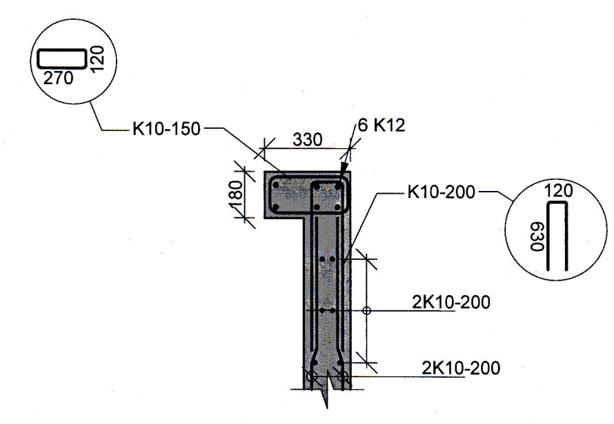
S1 Sula B_G-1.01 M 1:20
