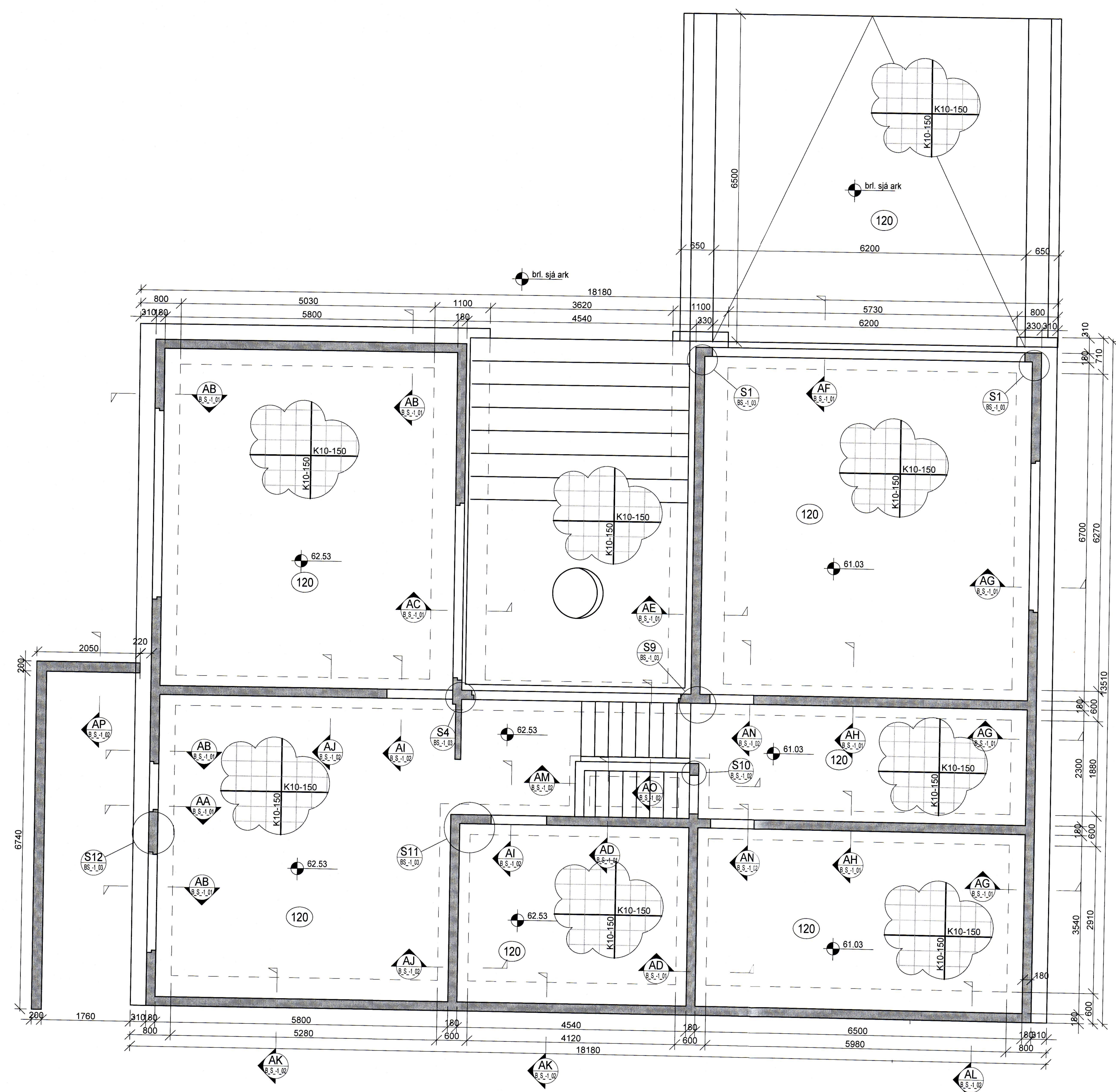
Grunnmynd M 1:50
