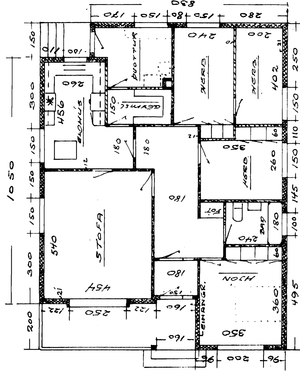
1. HÆÐ
