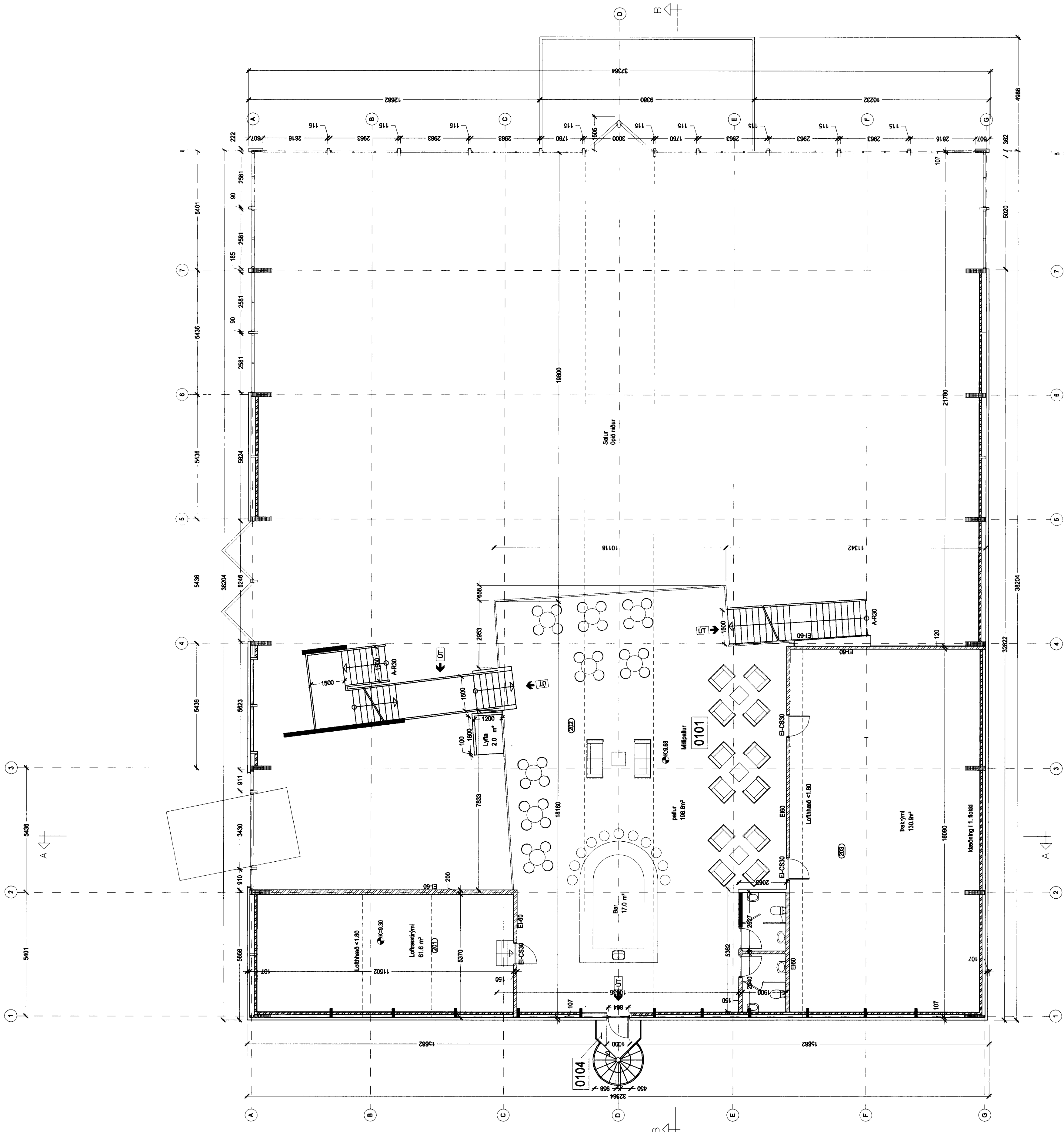
Grunnmynd millipalls, mkv. 1:100
