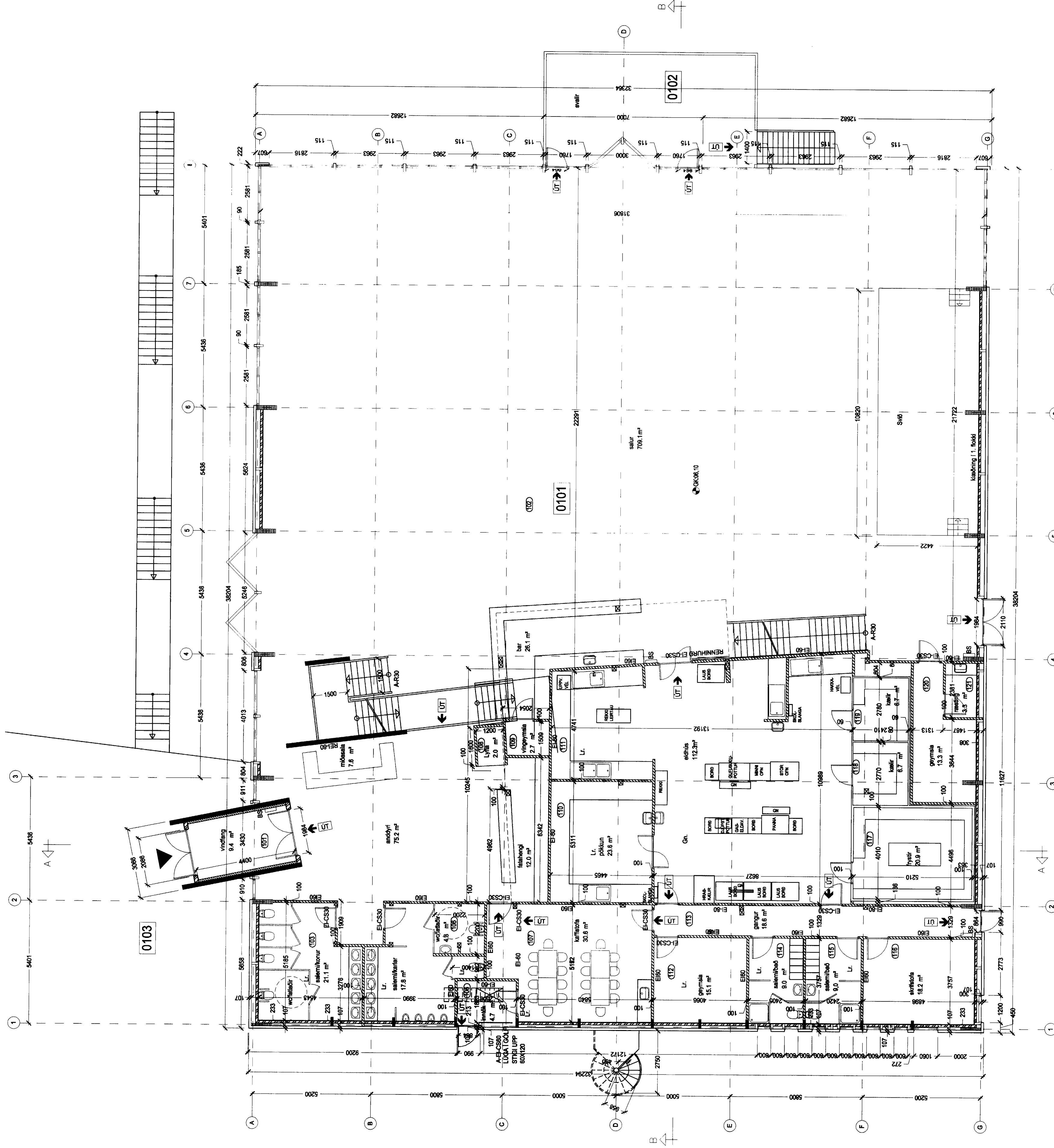
Grunnmynd 1. hæð, mkv. 1:100 Flاتمálm 1. hæðar er 1.236 m 2
