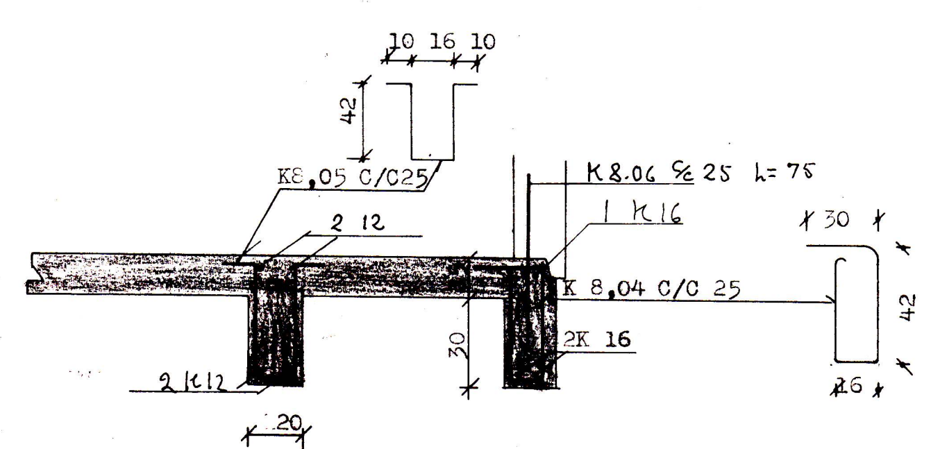
SNID E - E. 1:20.
