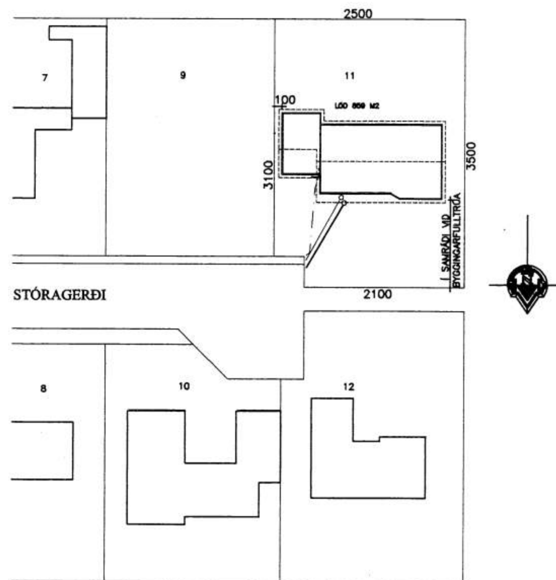
AFSTÖÐUMYND MKV. 1 : 500.
