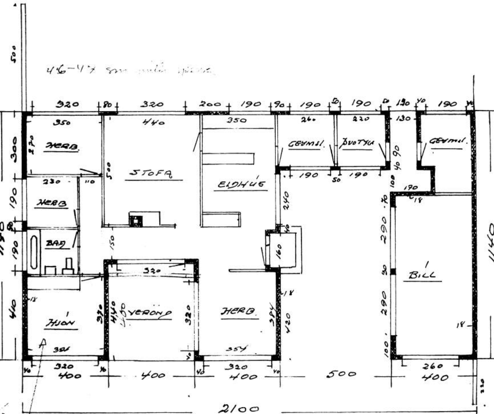
GRUNNFLÖTUR
