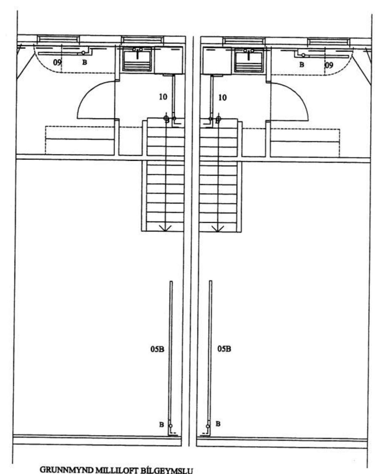
GRUNNMYND MILLILOFT BILGEYMSLU
