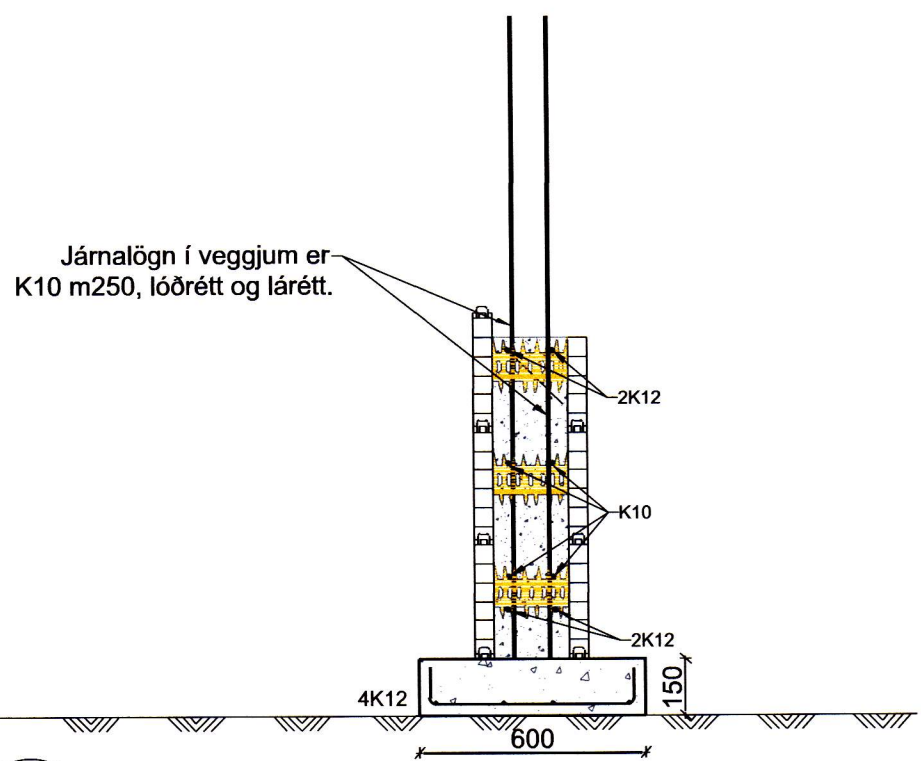
01 SNID í sökkulveggi 1:20
