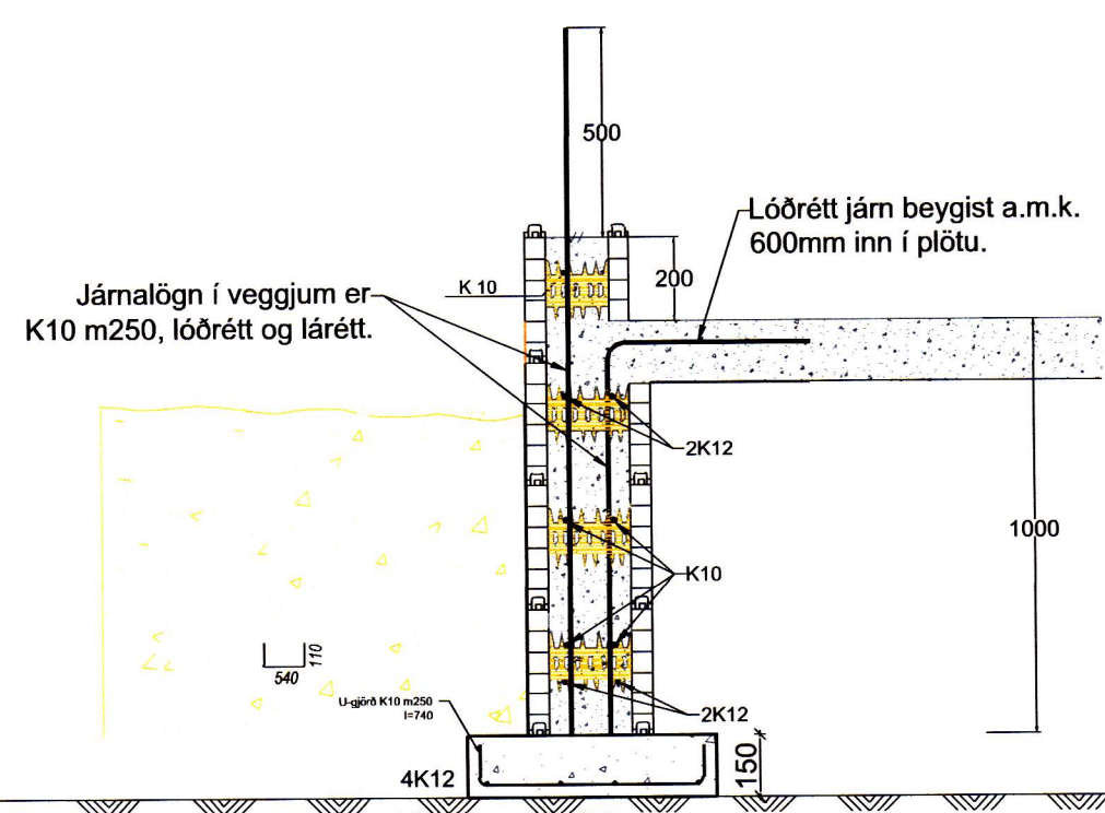
01 SNID fyrir botnplötu 1:20
