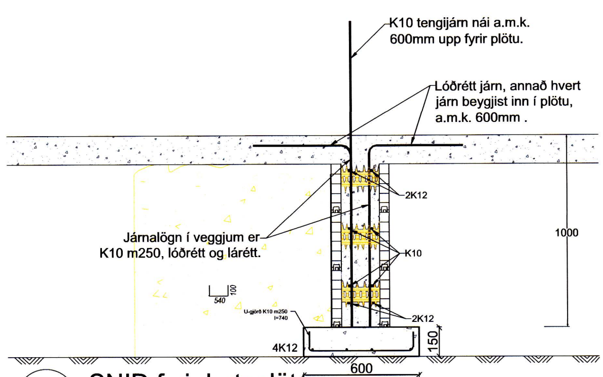
02 SNID fyrir botnplötu 1:20
