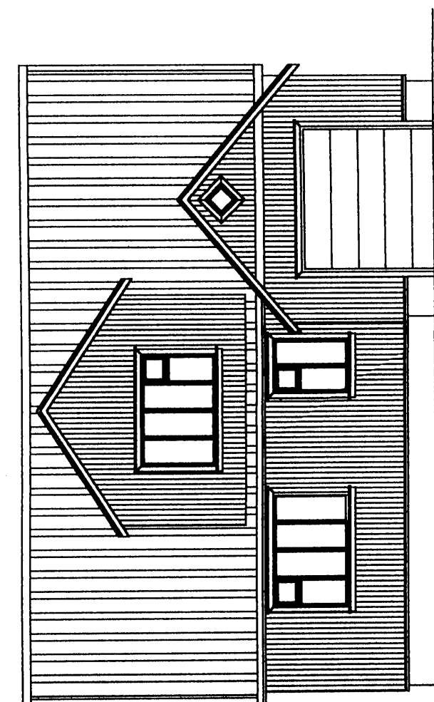
NORÐURHLÍÐ M=1:100
