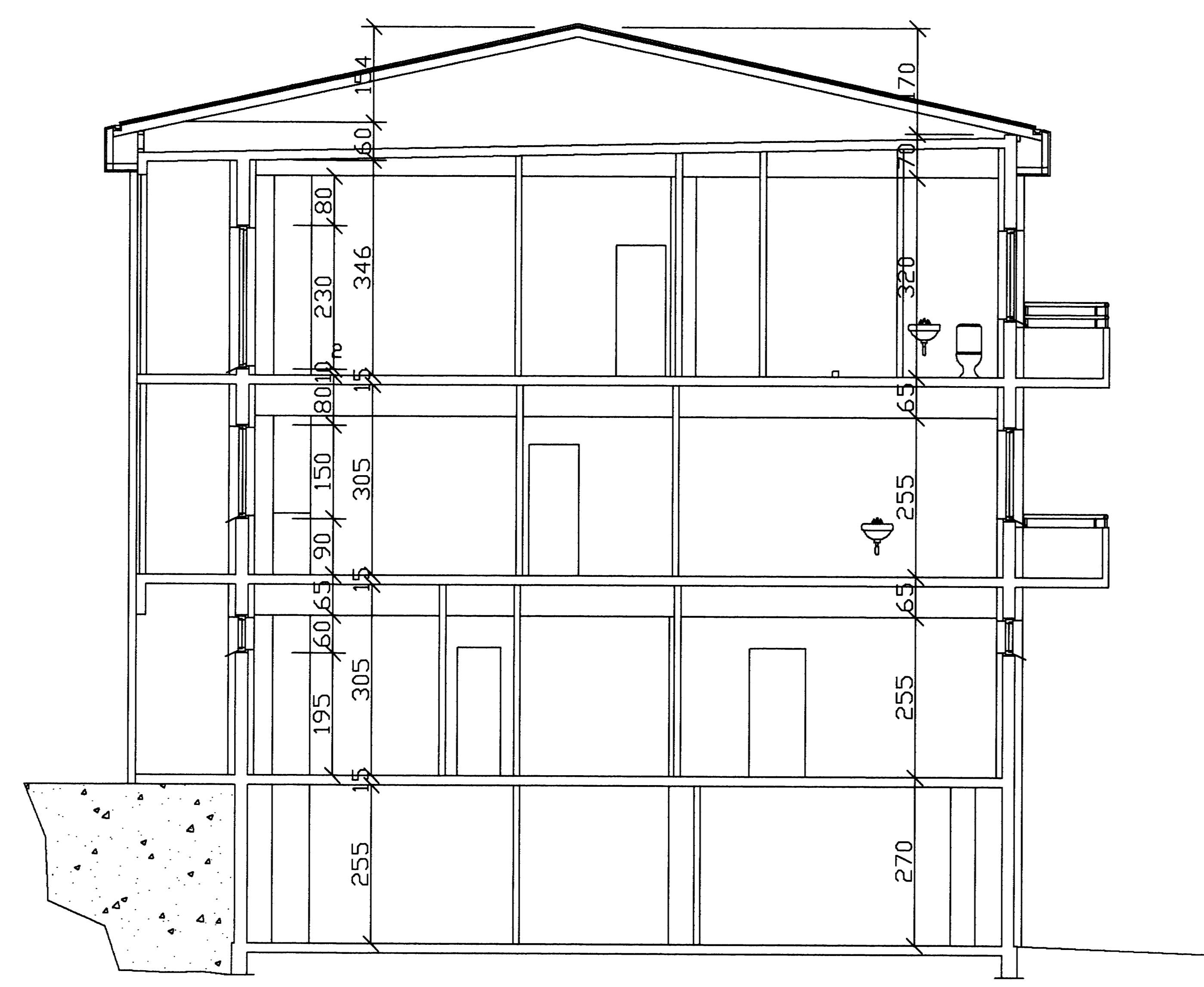
SNID A-A
