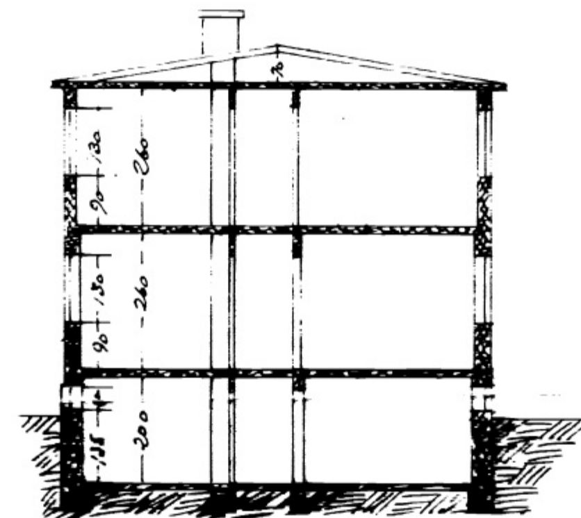
SKURÐUR
