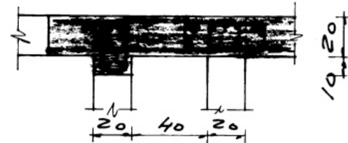
Súla S 1 1 : 20
