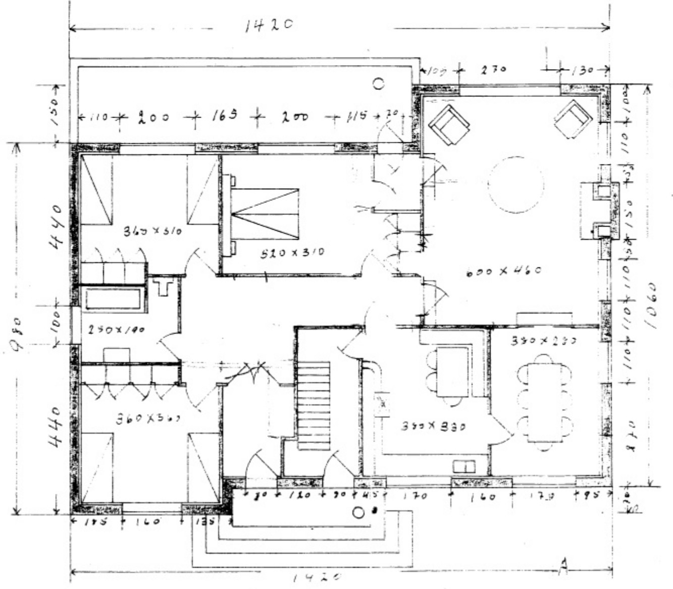
Grunnmynd
