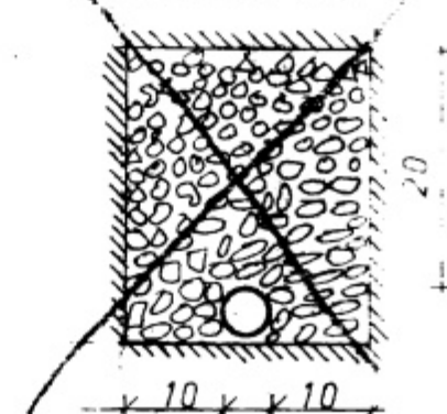
JARÐVATNSLÖGN RVERSNIÐ 1:10
