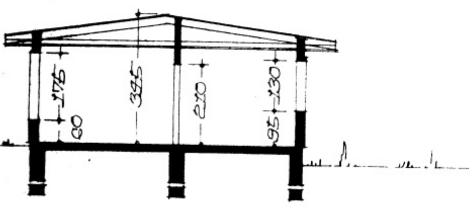
SKURÐUR B-B
