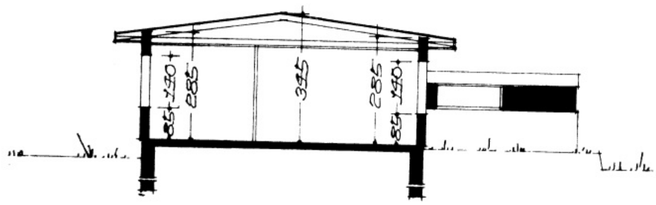
SKURÐUR A-A
