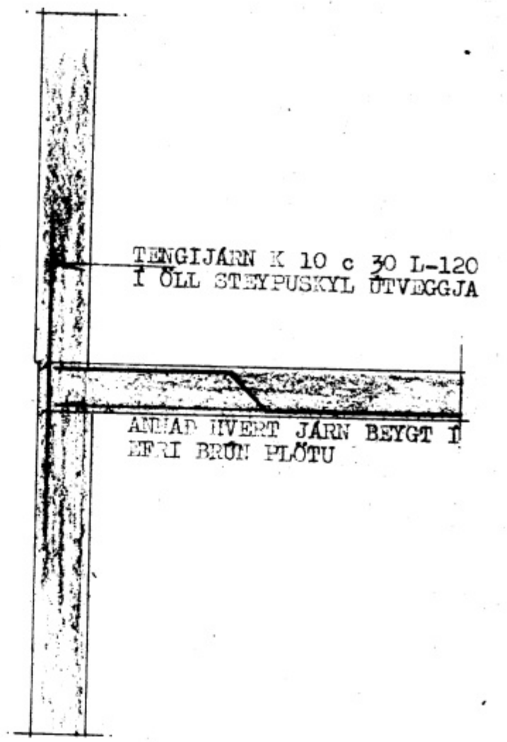
SNID I PLÖTU VÍÐ ÚTVEGG 1:20
