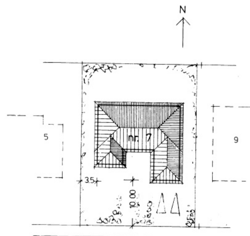
SMÁRAGATA AFSTÖÐUMYND 1:500
