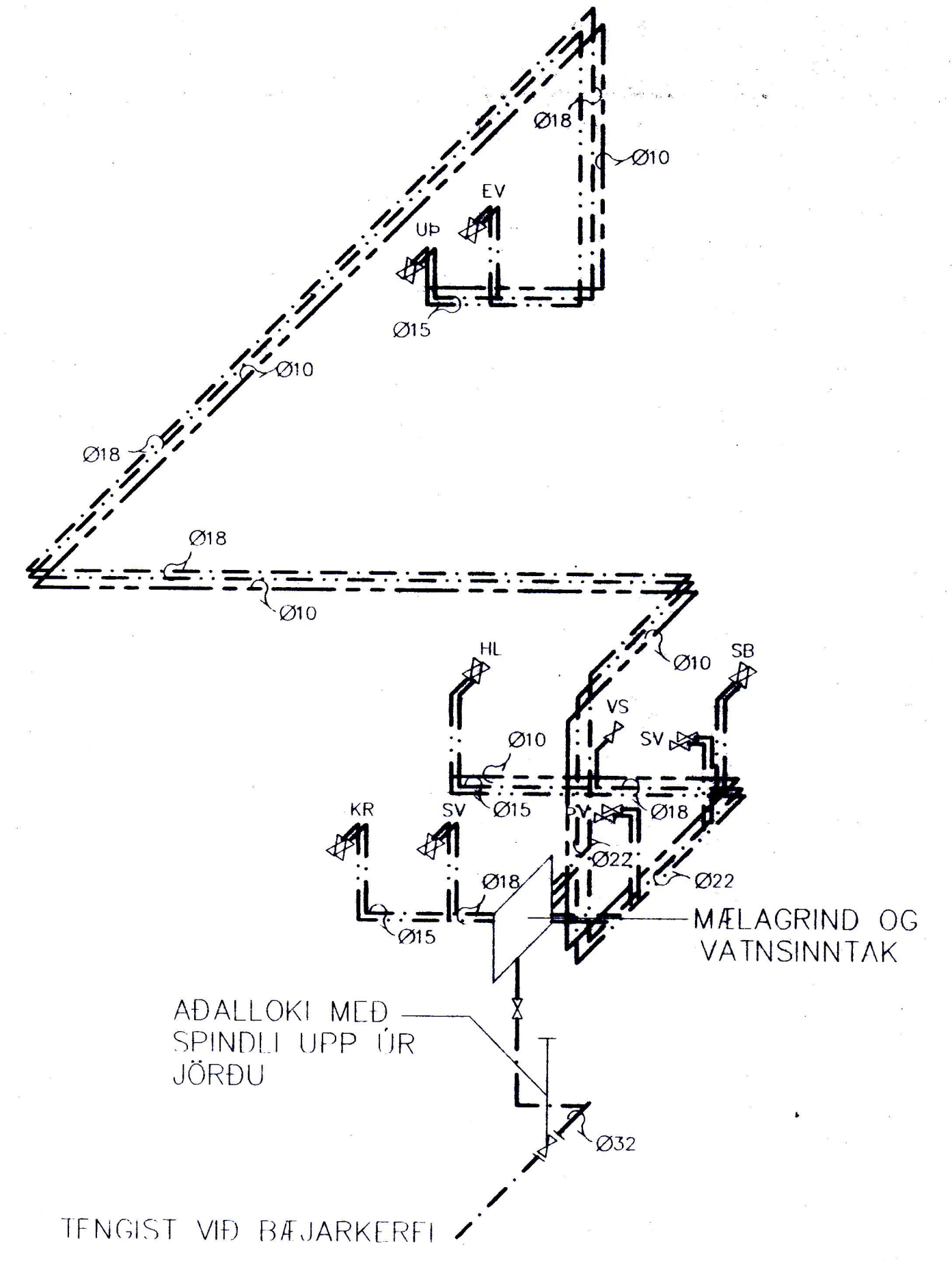
RÚMMYND VATNSLAGNA Mkv 1:50
