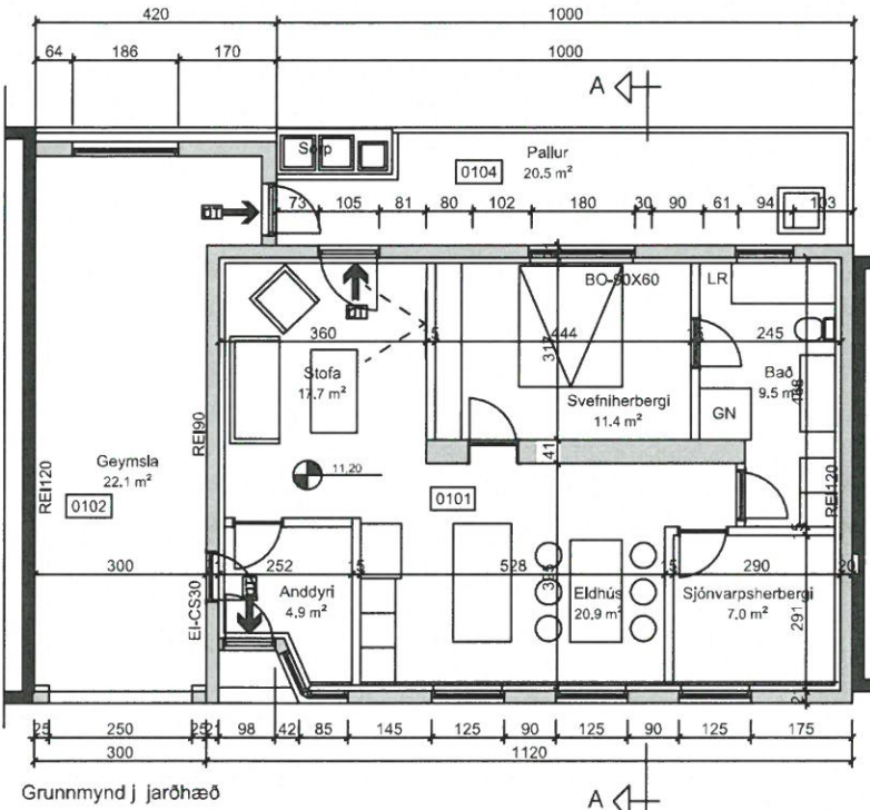
Grunnmynd | jarðhæð
