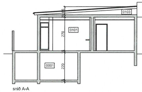
sníð A-A
