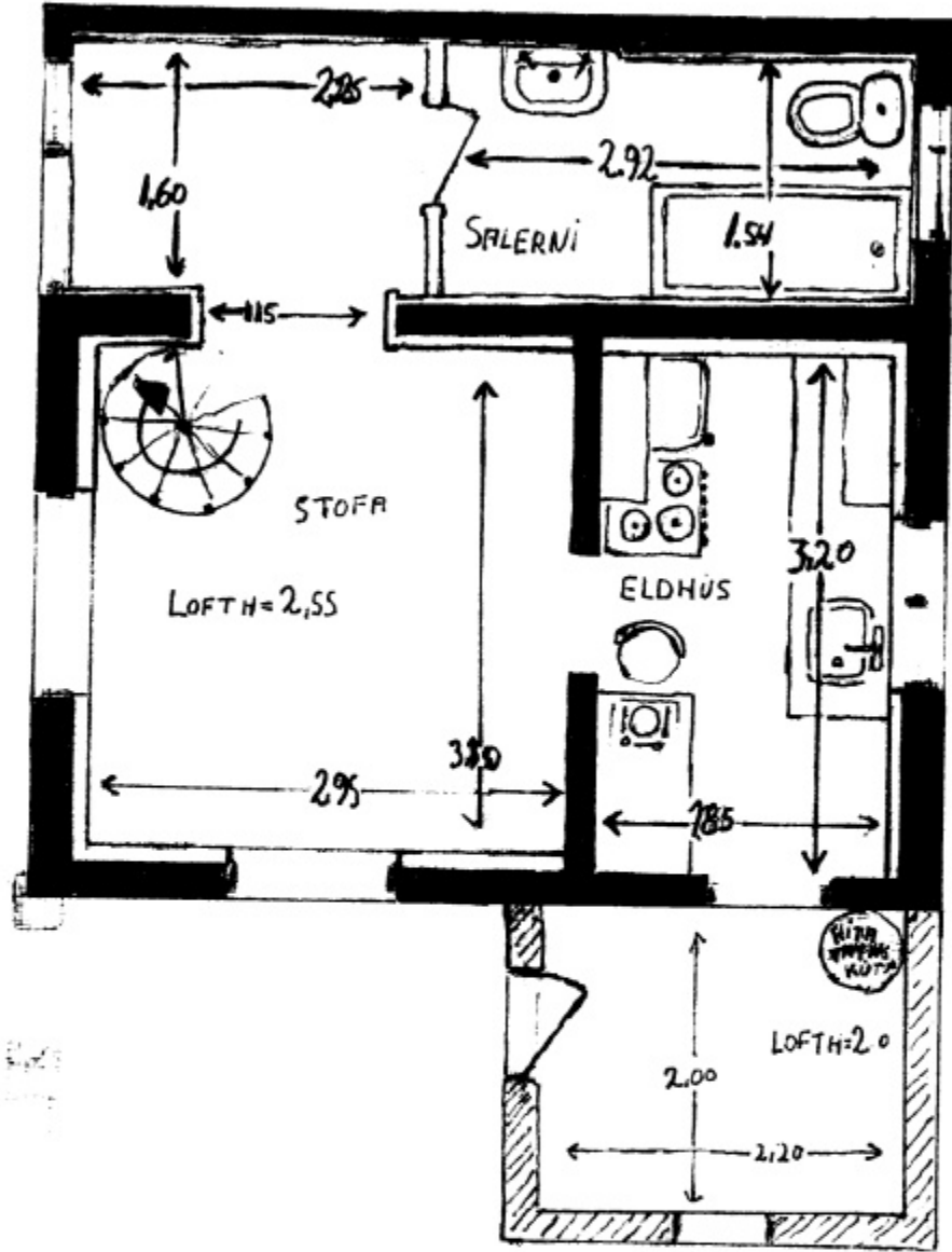
GRUNNMYND 1 HÆÐ
