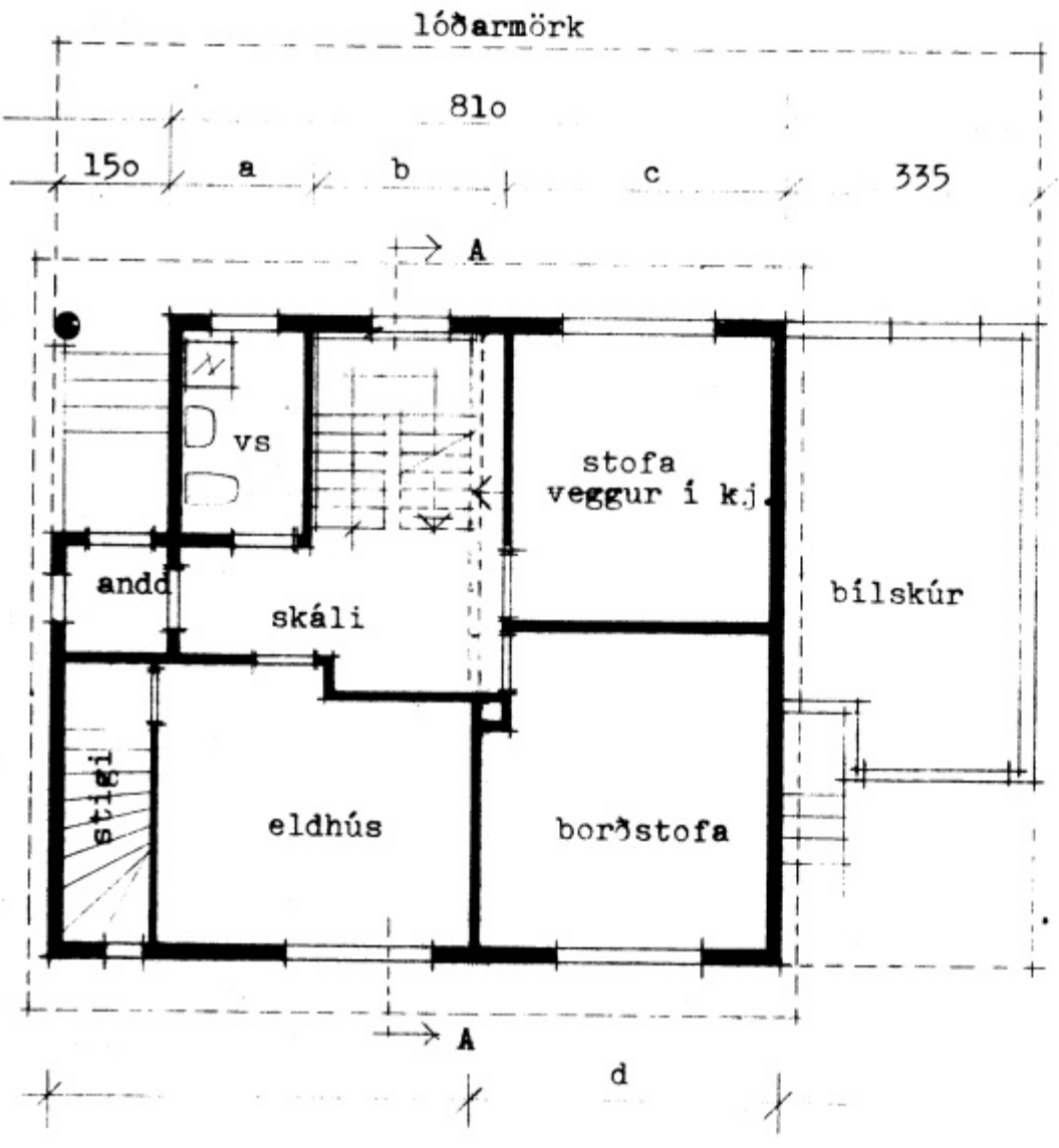
GRUNNMYND 1. HÆÐ
