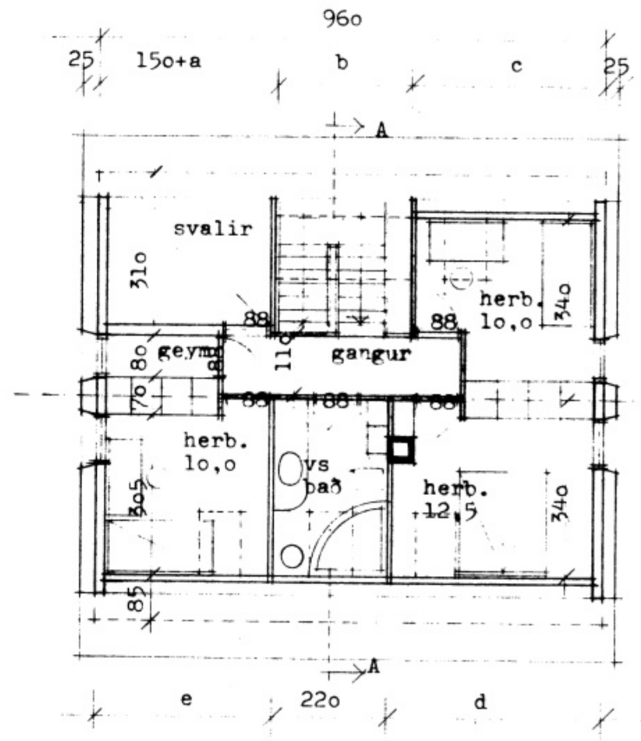
GRUNNMYND RISHÆÐ
