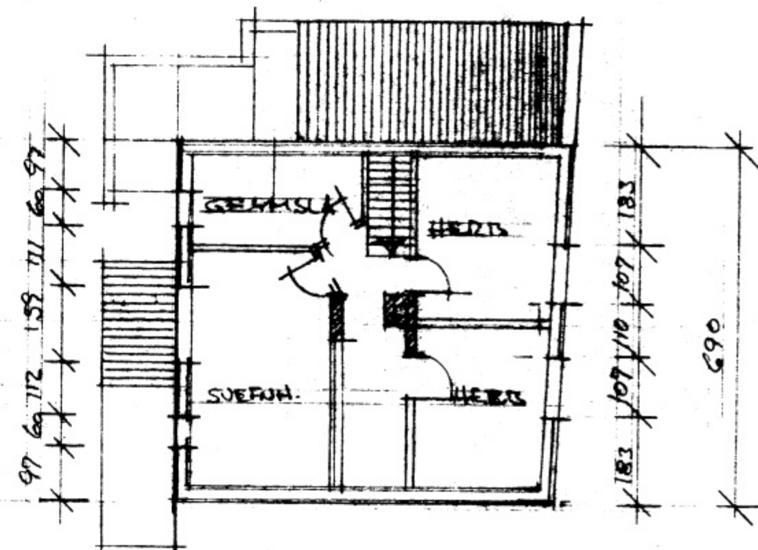
GRUNNMYND 2 HÆÐ
