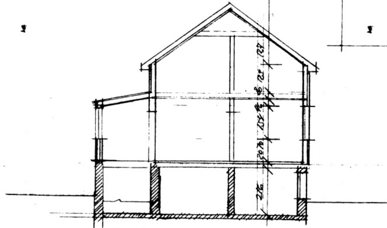
SNIT A-A 1:100
