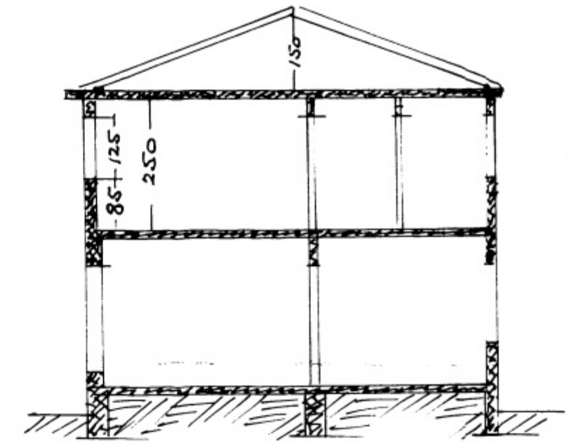
SKURÐUR
