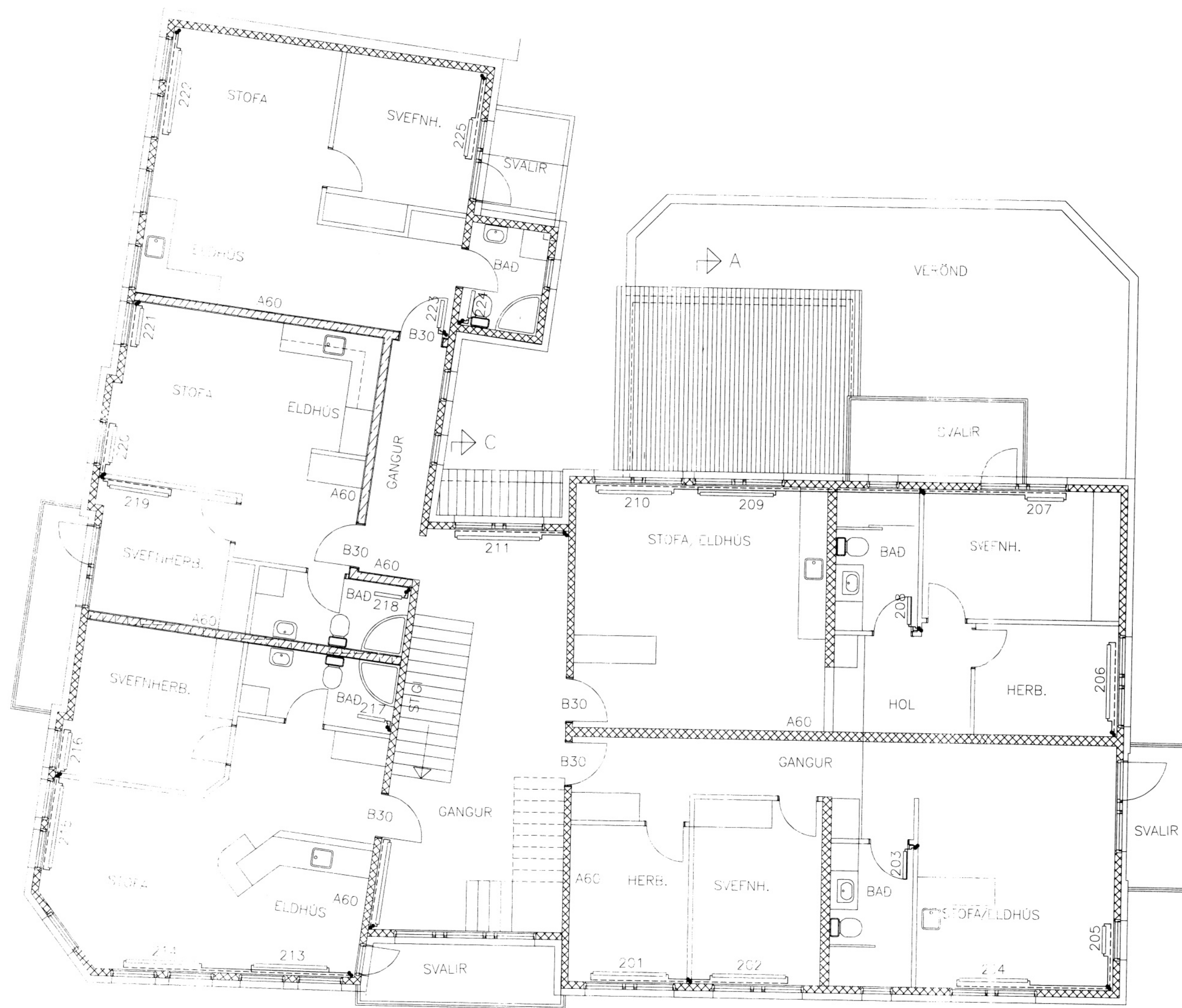
GRUNNMYND 2. HÆÐ
