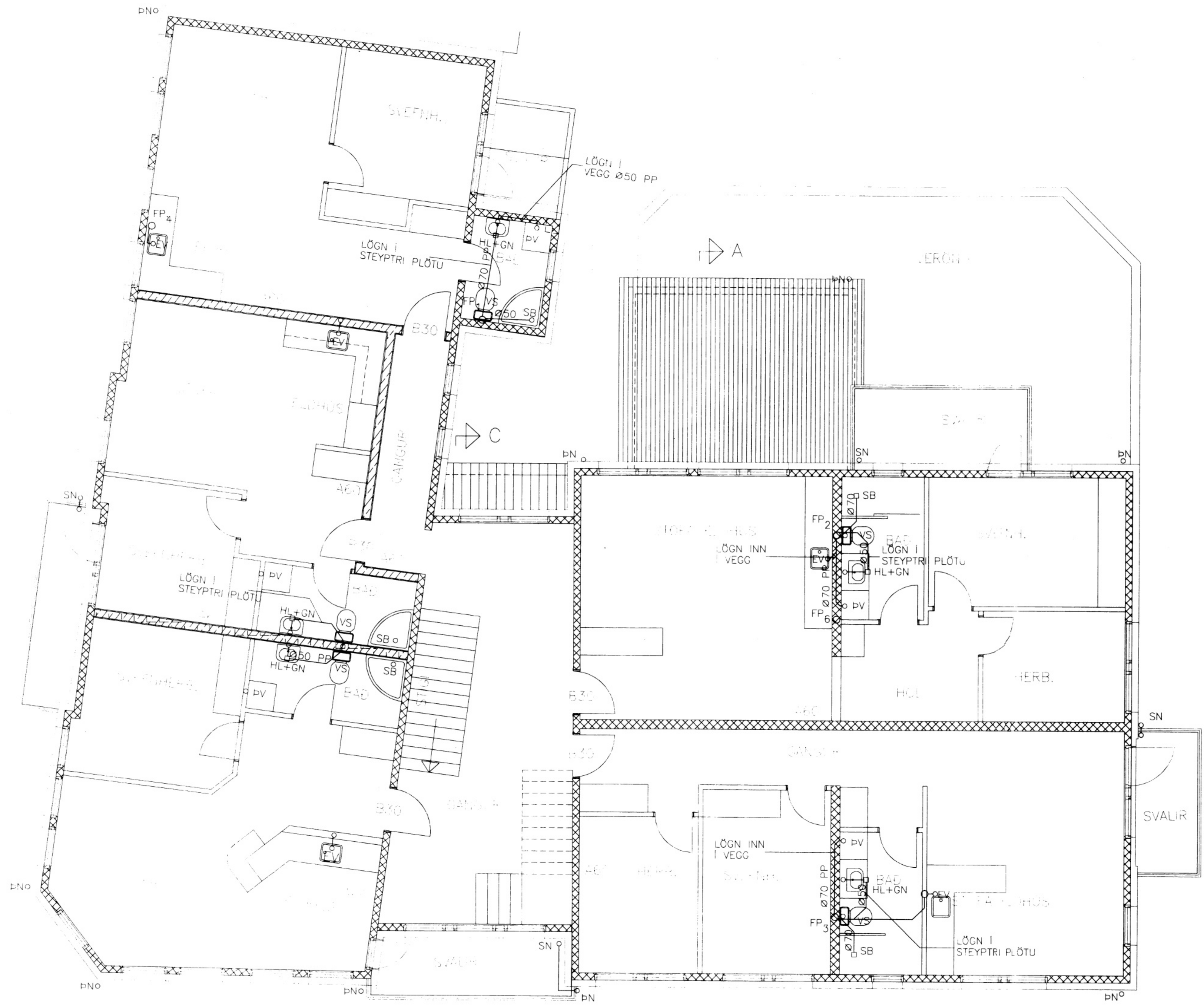
GRUNNMYND 2. HÆÐ
