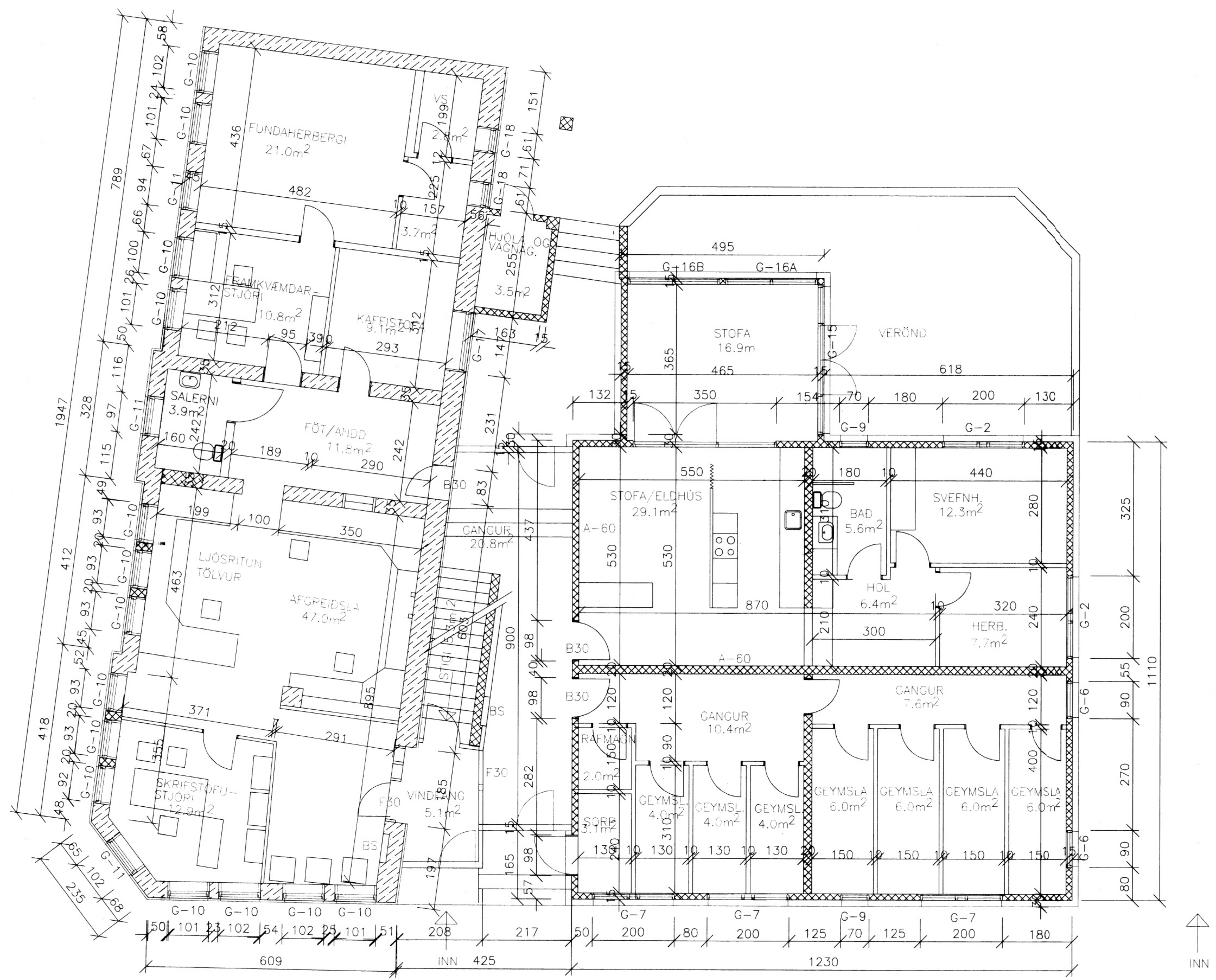
GRUNNMYND 1. HÆÐ
