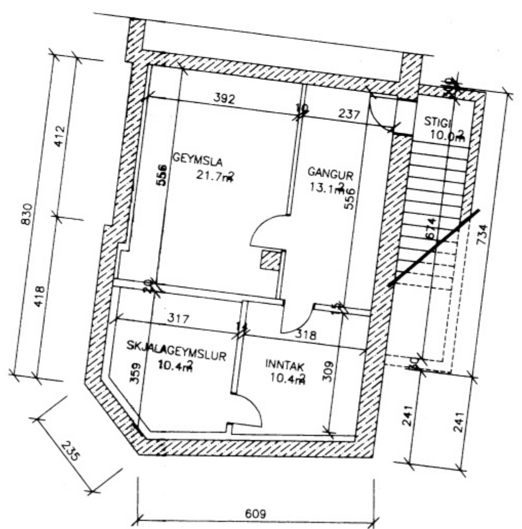
GRUNNMYND KJALLARI M=1:100
