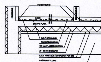
SNIÐ Í GÓLF Mkv. 1:20
