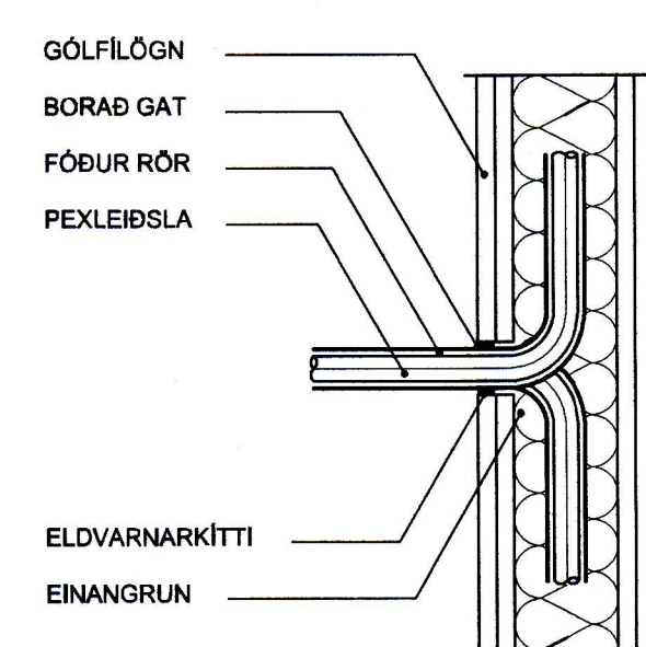
BRUNAÞÉTTING Á PEXLEIÐSLU Í FÓÐURRÖRI Í GEGNUM KLÆDNINGU
