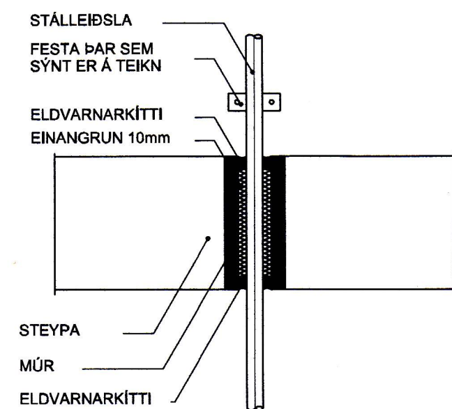
FRÁGANGUR Á STÁLLEIÐSLU GEGNUM STEYPT GÓLF
