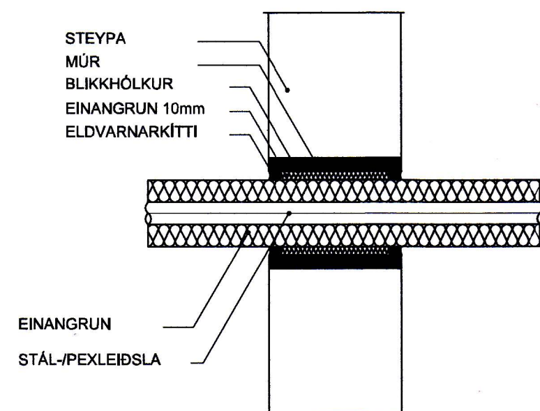
FRÁGANGUR Á STÁL-/PEXLEIÐSLU GEGNUM STEYPTAN VEGG
