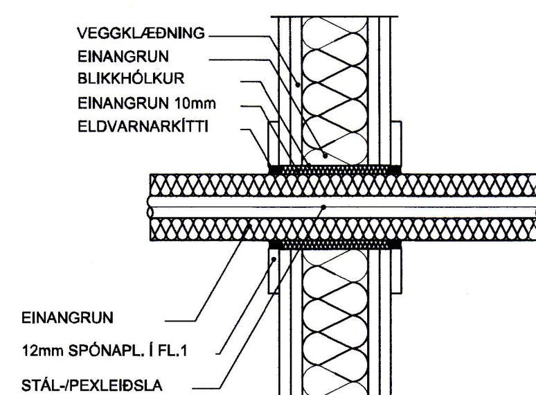
FRÁGANGUR Á STÁL-/PEXLEIÐSLU GEGNUM LÉTTAN VEGG
