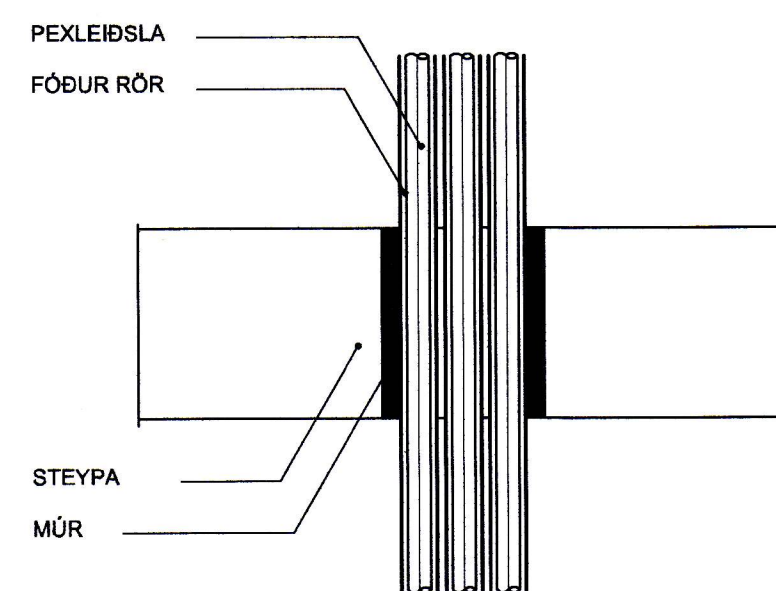
FRÁGANGUR Á PEXLEIÐSLU GEGNUM STEYPT GÓLF
