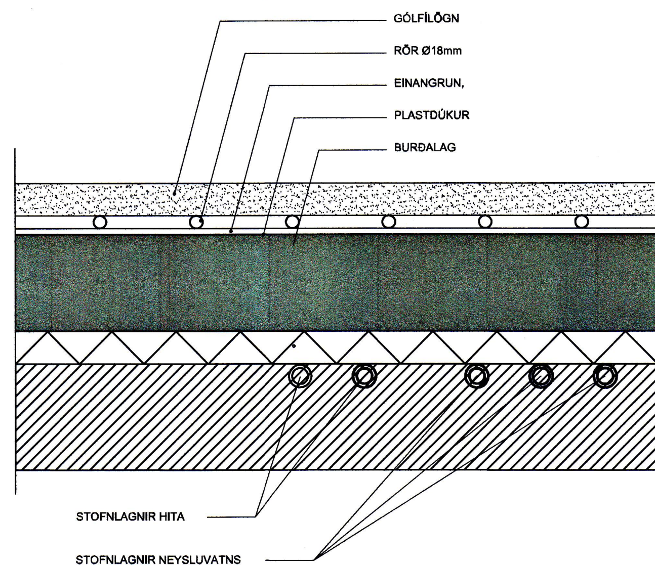
FRÁGANGUR LAGNA Í GÓLFI
