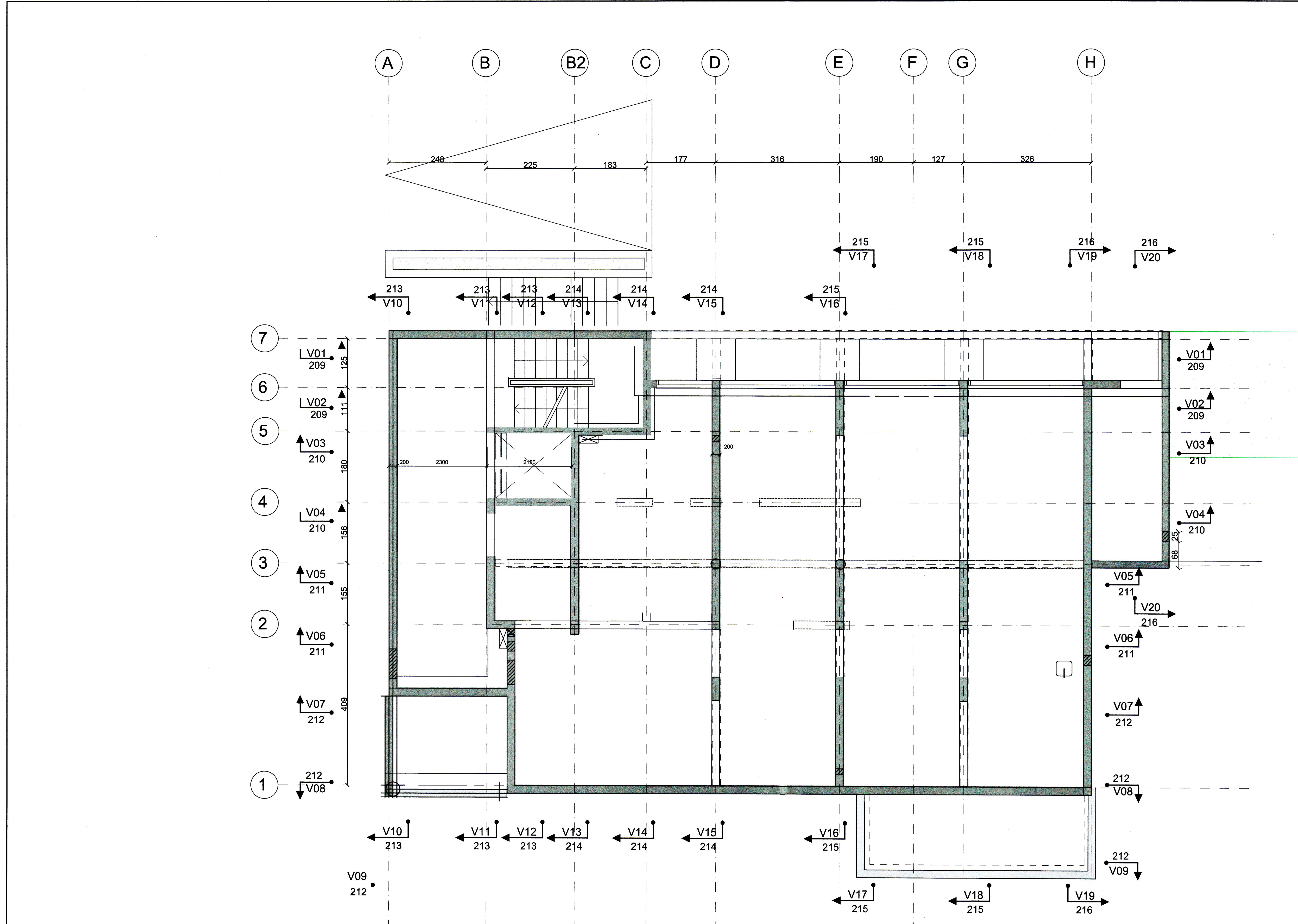
GRUNNMYND PLATA YFIR KJALLARA 1:50
