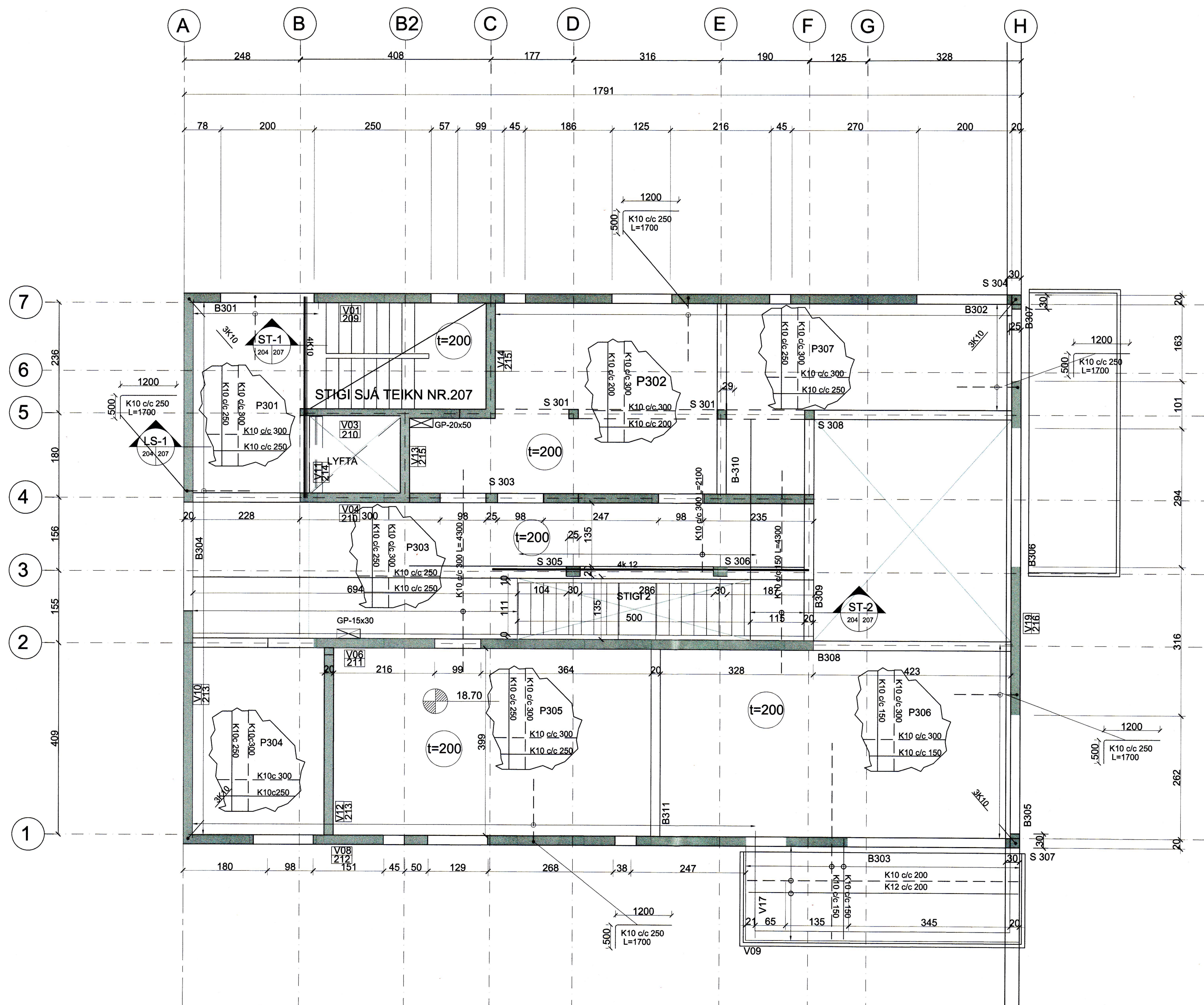
GRUNNMYND PLATA YFIR 2. HÆÐ 1:50
