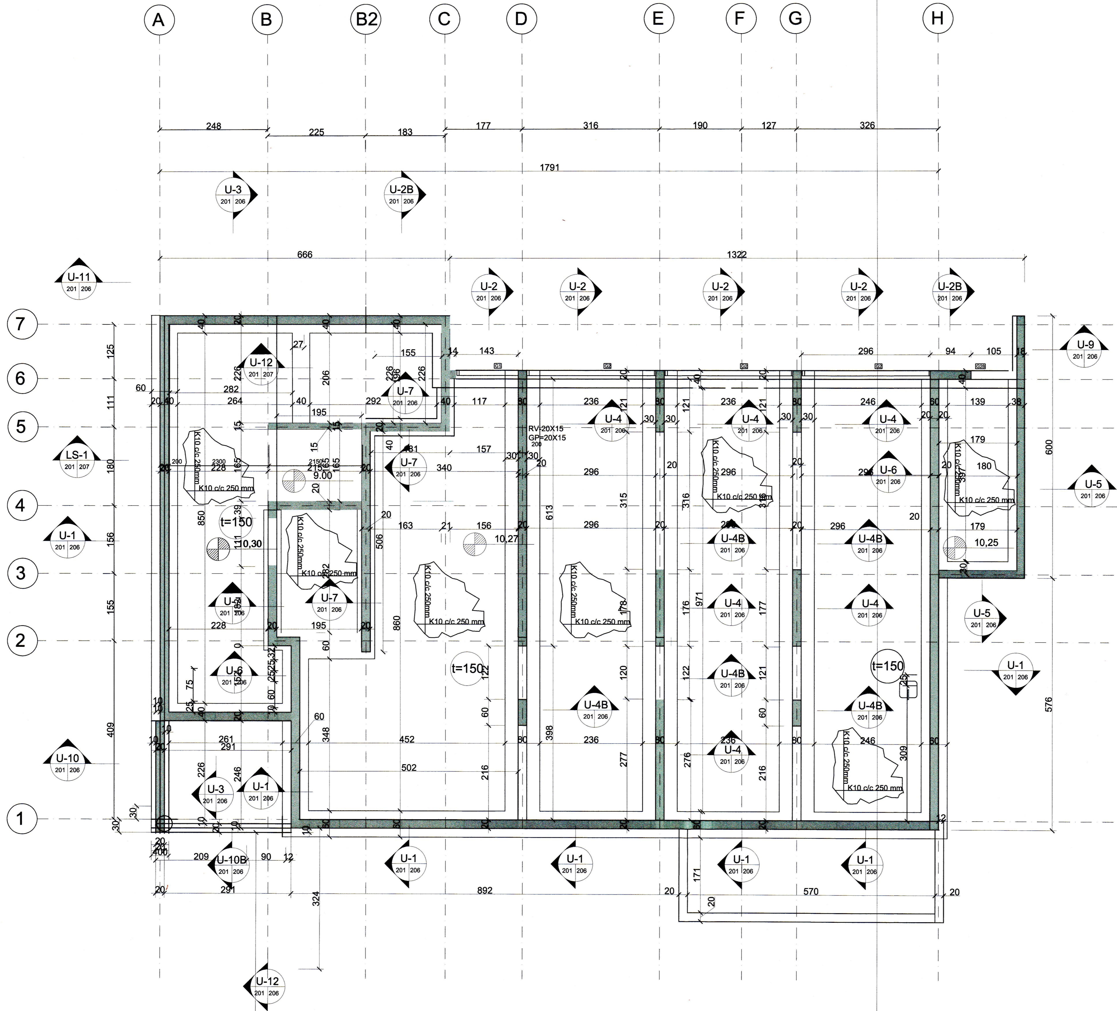
GRUNNMÝND UNDIRSTÖÐUR 1:50
