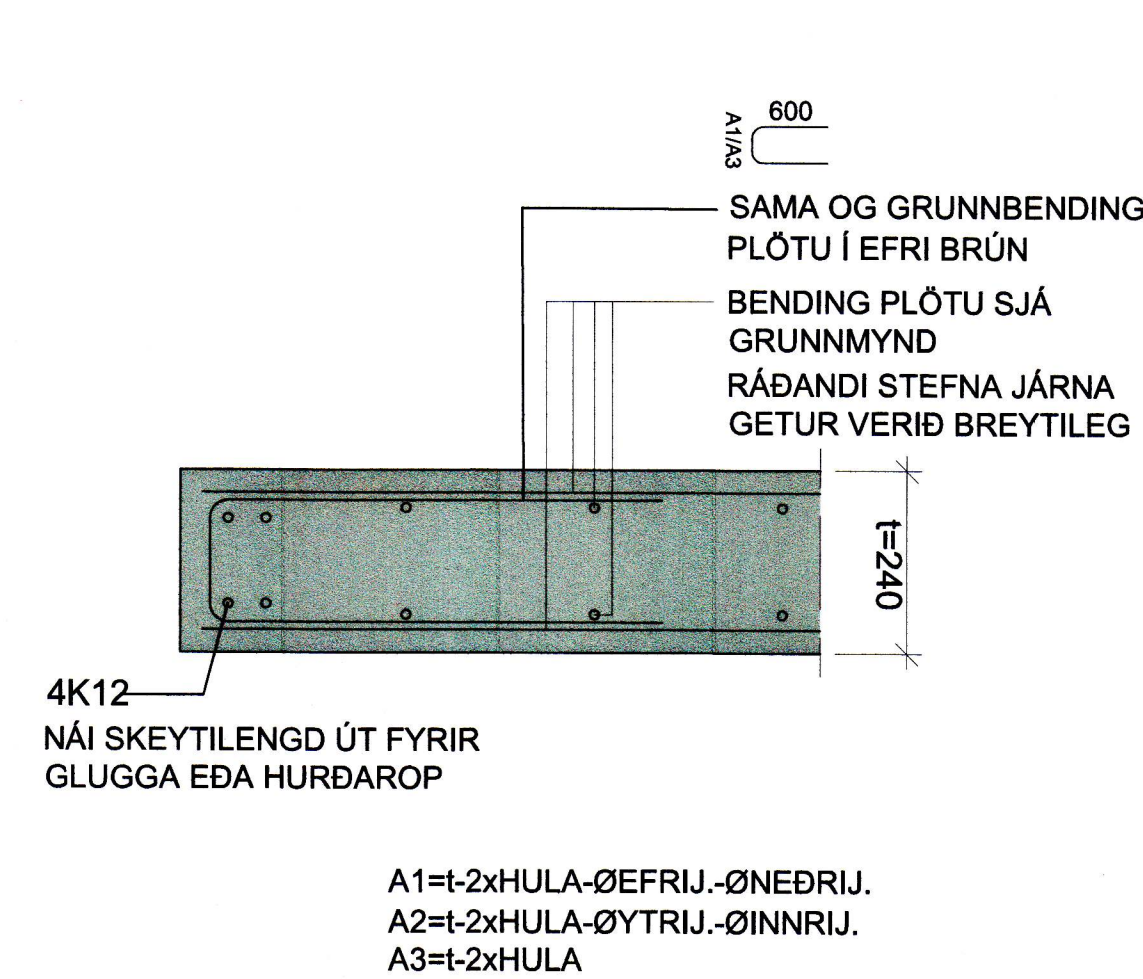
LÓÐRÉTT SNIÐ M1:10: STAÐSTEYPT PLATA AÐ ÚTVEGG ÞAR SEM EKKI ER BITI
