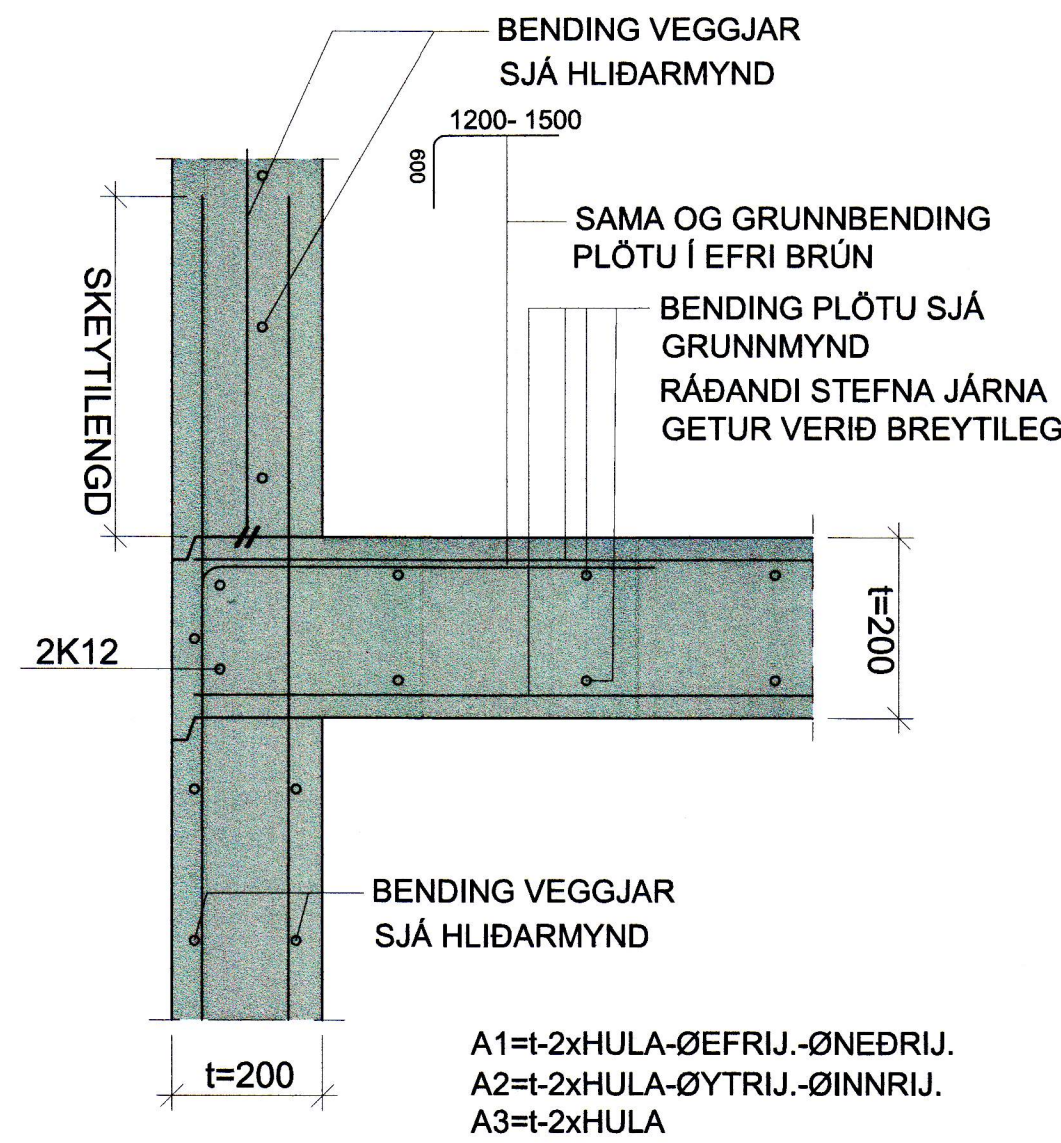
LÓÐRÉTT SNIÐ M1:10: STAÐSTEYPT PLATA AÐ ÚTVEGG YFIR KJALLARA
