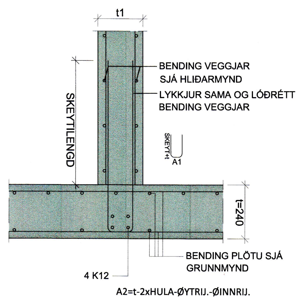
LÓÐRÉTT SNIÐ M1:10: TENGINN VEGGUR YFIR PLÖTU
