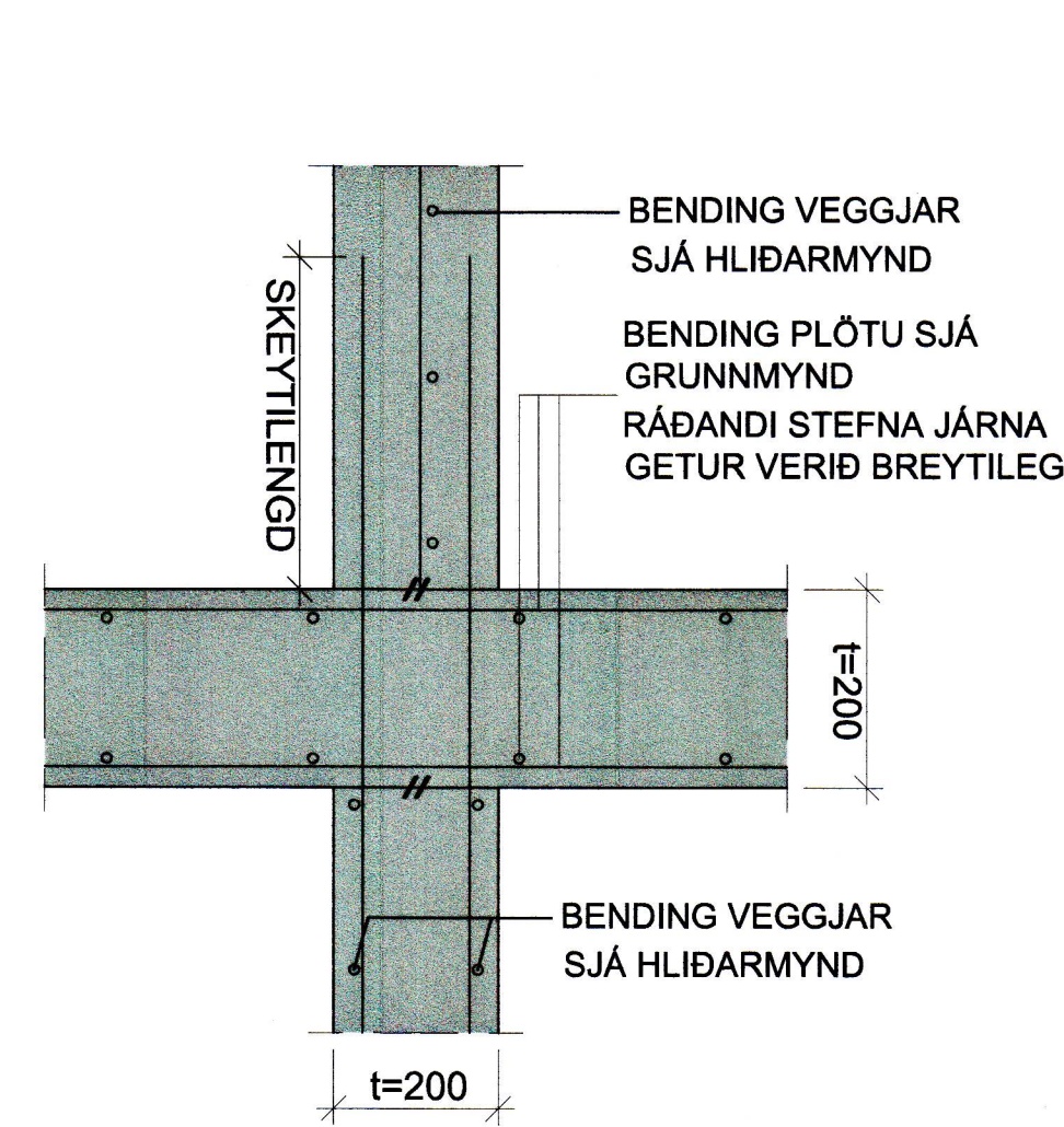
LÓÐRÉTT SNIÐ M1:10: STAÐSTEYPT PLATA AÐ INNVEGG
