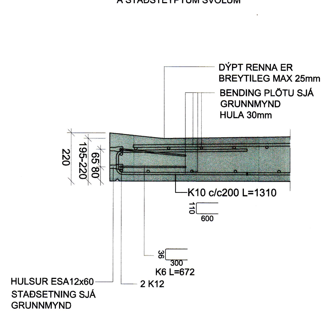
LÓÐRÉTT SNIÐ M1:10: INNSTEYPT FESTING FYRIR SVALAHANDRÍÐ Á STAÐSTEYPTUM SVÖLUM
