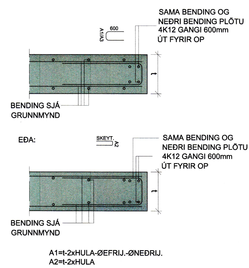
LÓÐRÉTT SNIÐ M1:10: FRÁGANGUR Á PLÖTU VIÐ OP
