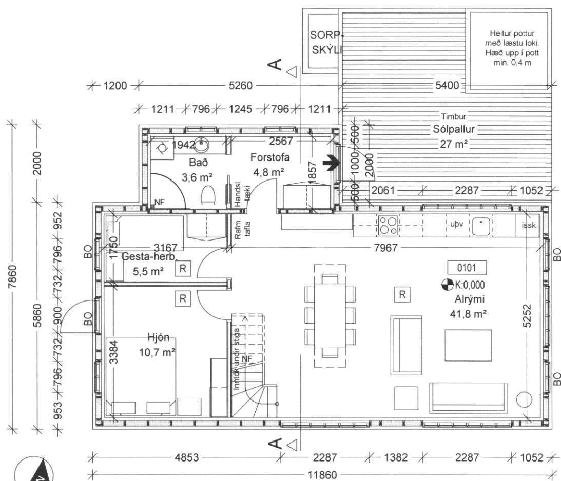
GRUNNMYND 1H 1:100
