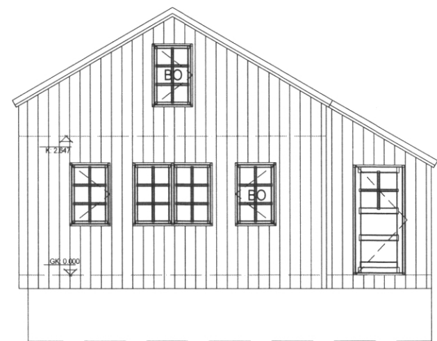
ÚTLIT MÓTI NORÐUR 1:100
