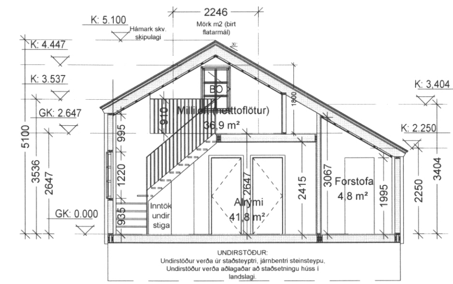
SNEIÐING A-A 1:100
