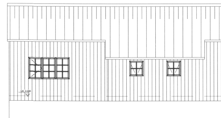
ÚTLIT MÓTI VESTUR 1:100
