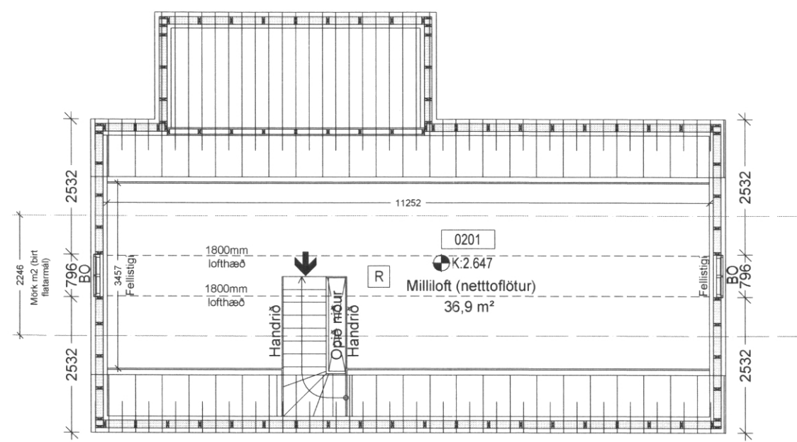
GRUNNMYND 2H 1:100
