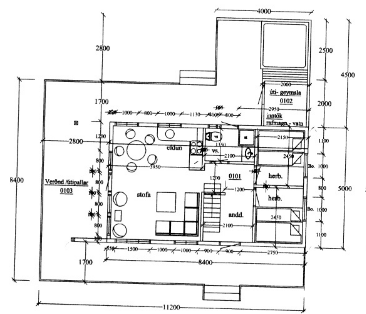
Grunnmynd 1. Hæð M 1:100
