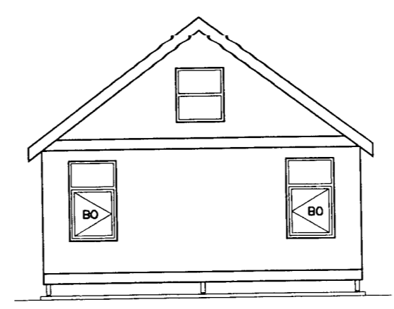
AUSTLÆG-HLID M 1:100
