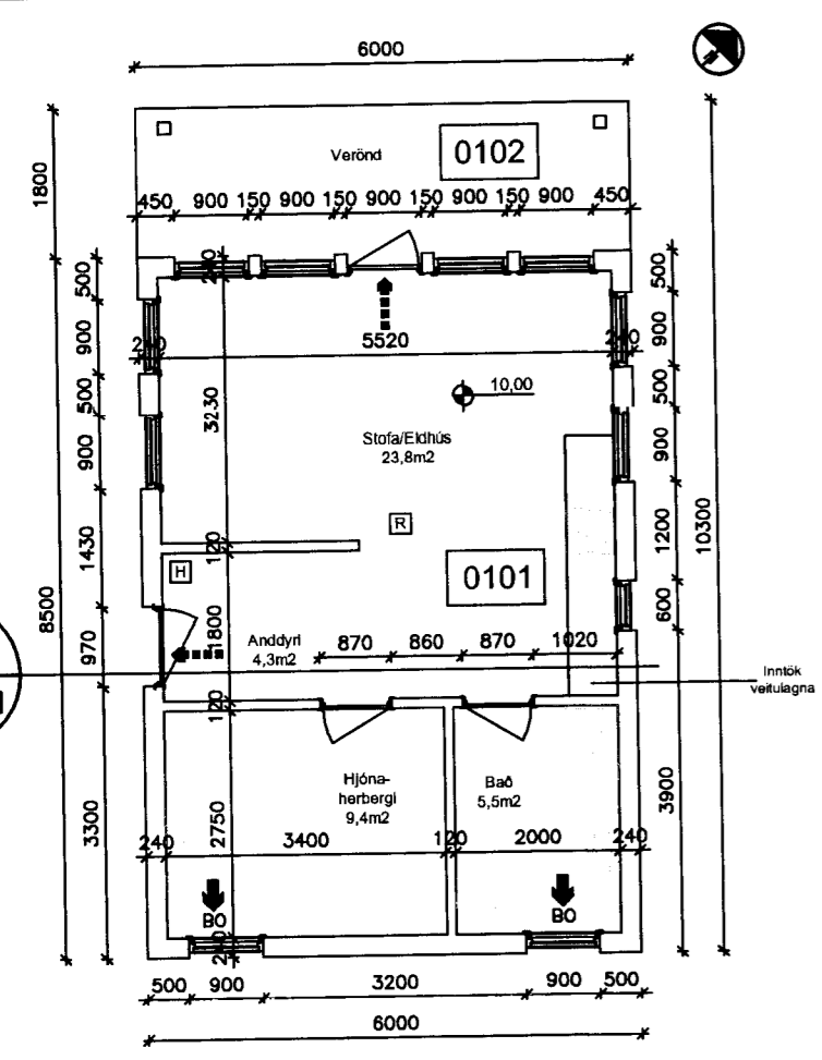
GRUNNMYND-0101 M 1:100
