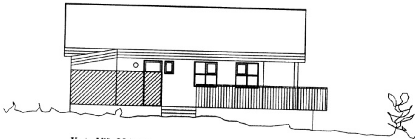
Vesturhlíð M 1:100
