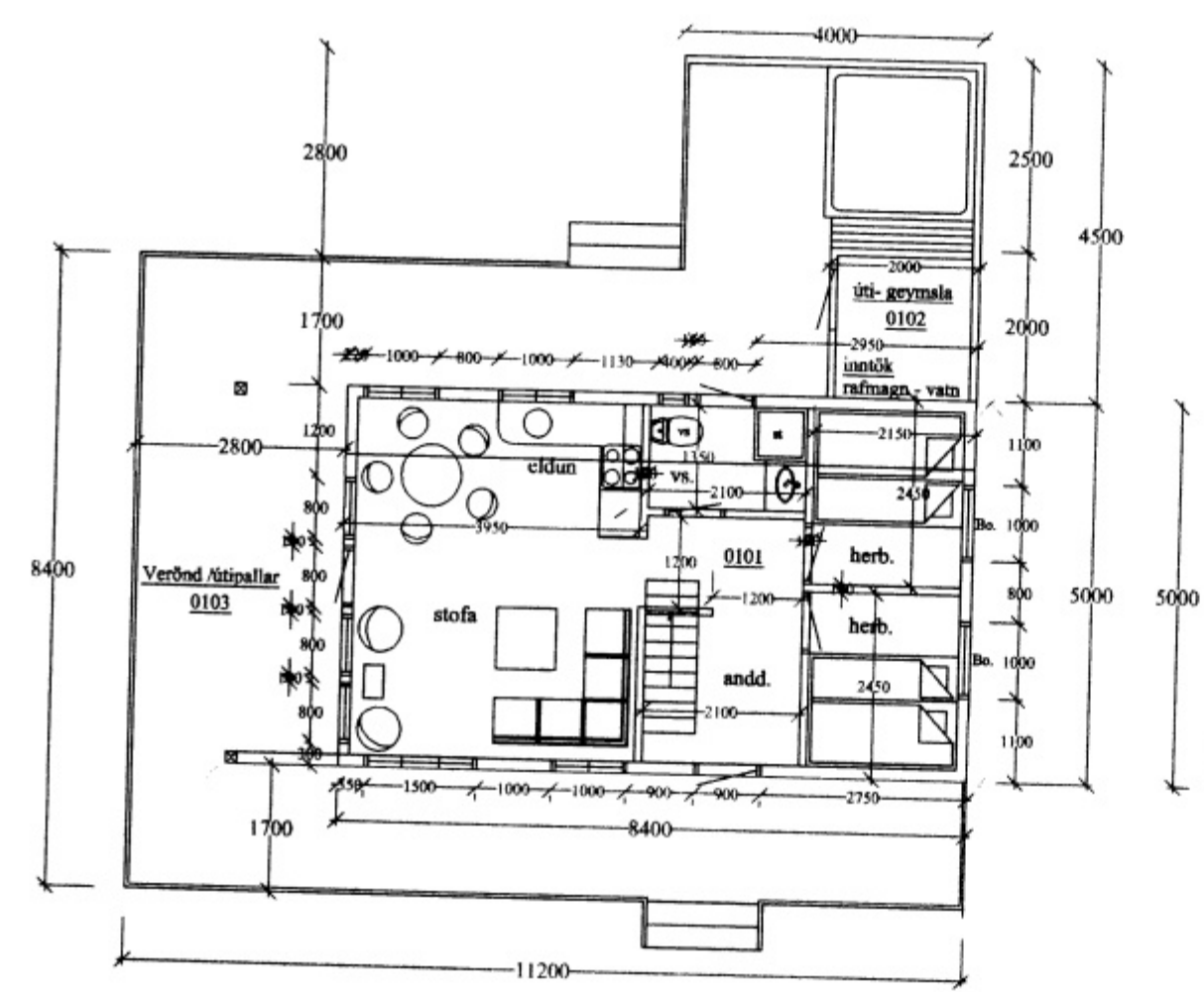
Grunnmynd 1. Hæð M 1:100
