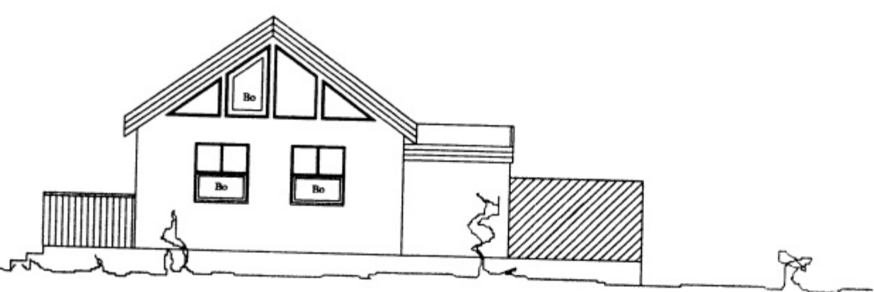
Norðurhlíð M 1:100
