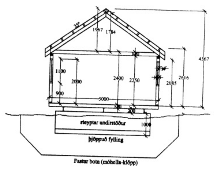
Þversnið M 1:100
