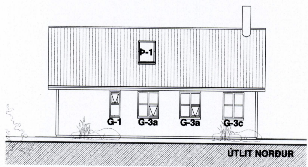
3. Gluggayfirlit 1:50
