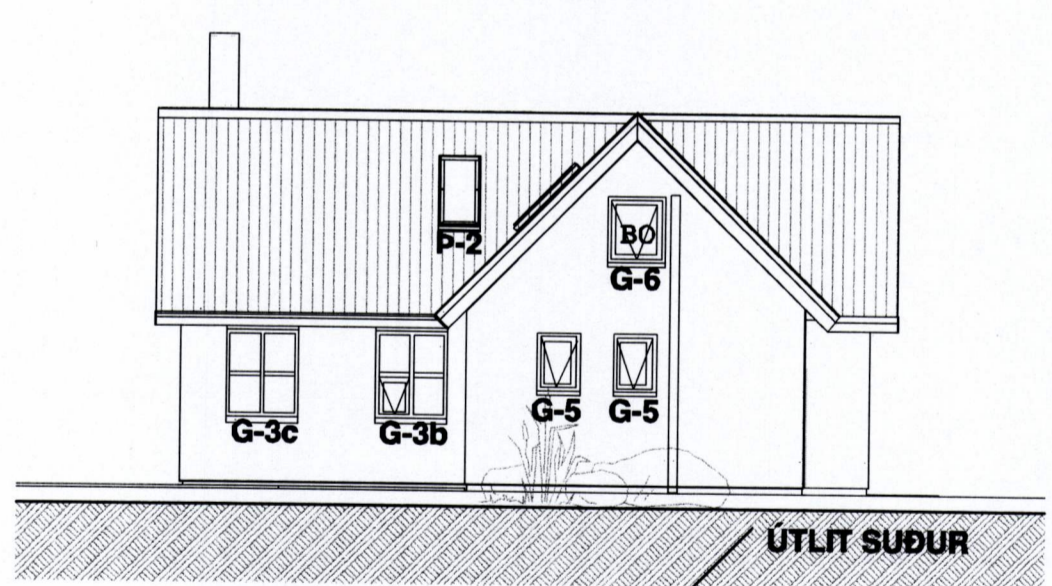
3. Gluggayfirlit 1:50
