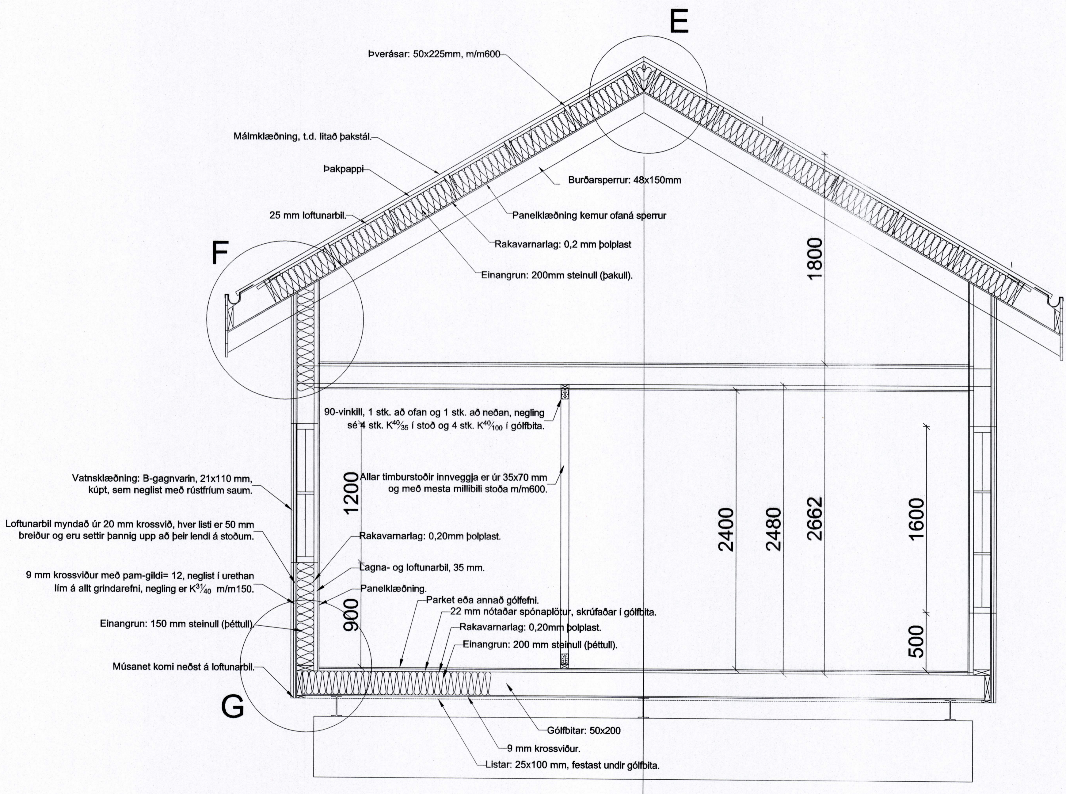
Kennisnið í sumarbústað með efnisskýringum, mkv.= 1:20.
