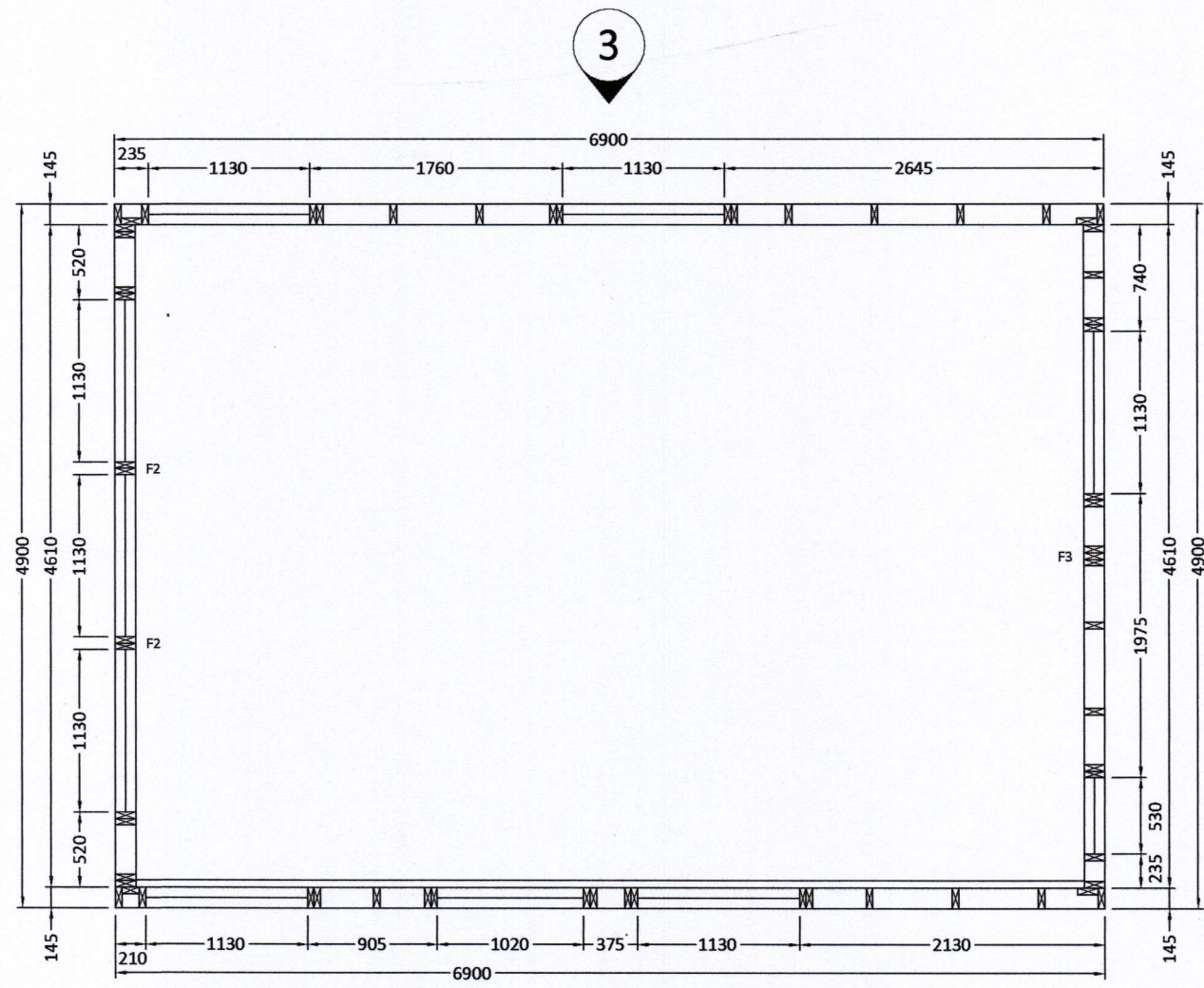
GRUNNMYND VEGGJA MVK. 1:50
