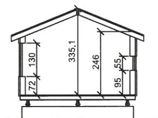
sneiðing mkv 1:100
