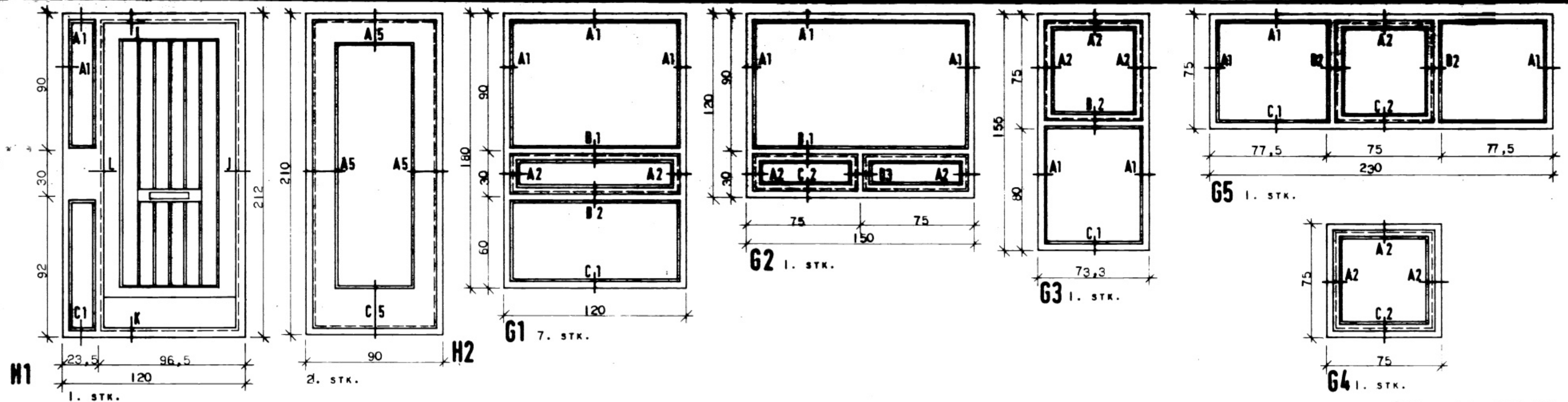
ÍSTEYPTIR GLUGGAR Á NEÐRI HÆÐ.
