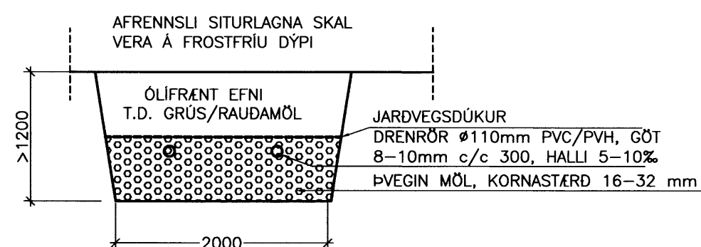
SITURLÖGN, SNID A-A Mkv. 1:50
