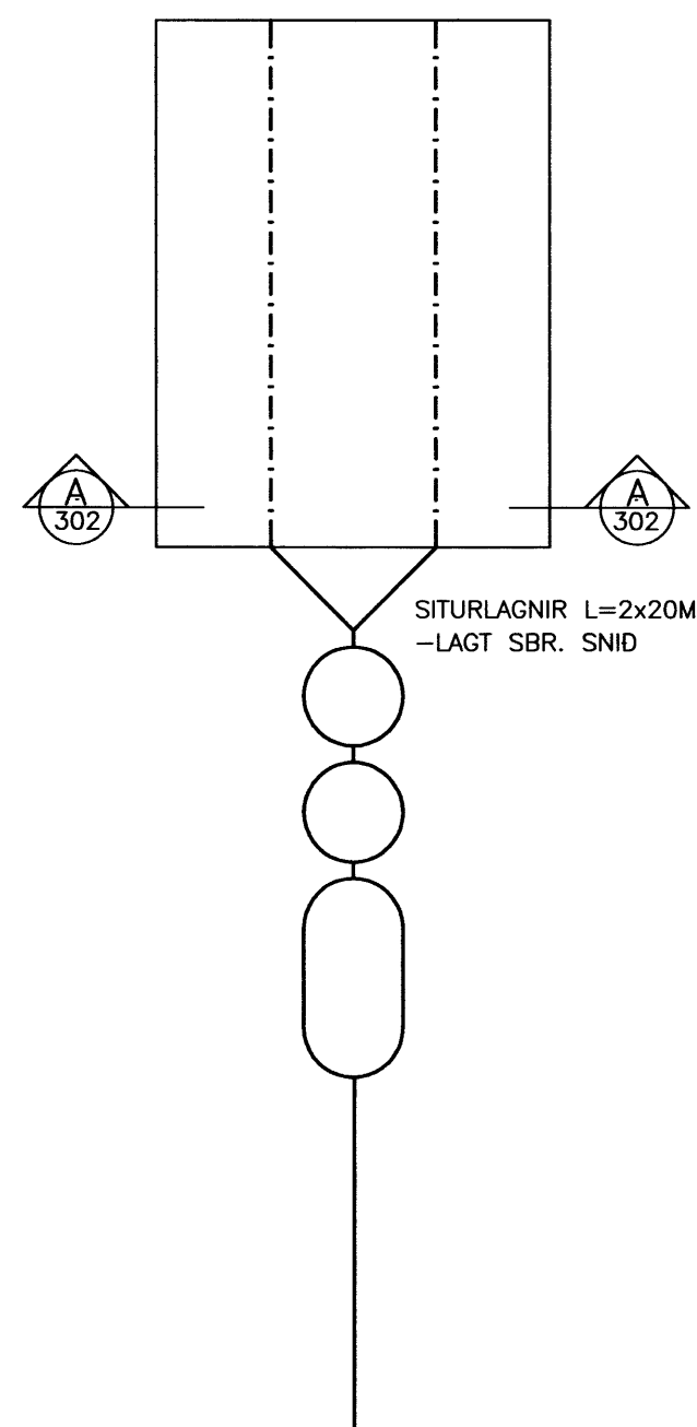
ROTÞRÓ GRUNNMYND Mkv. 1:50
