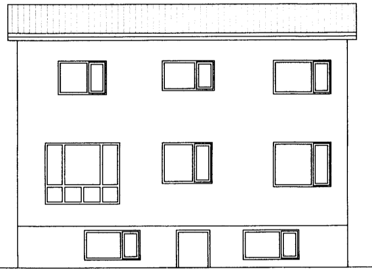
NORÐUHLIÐ 1:100
