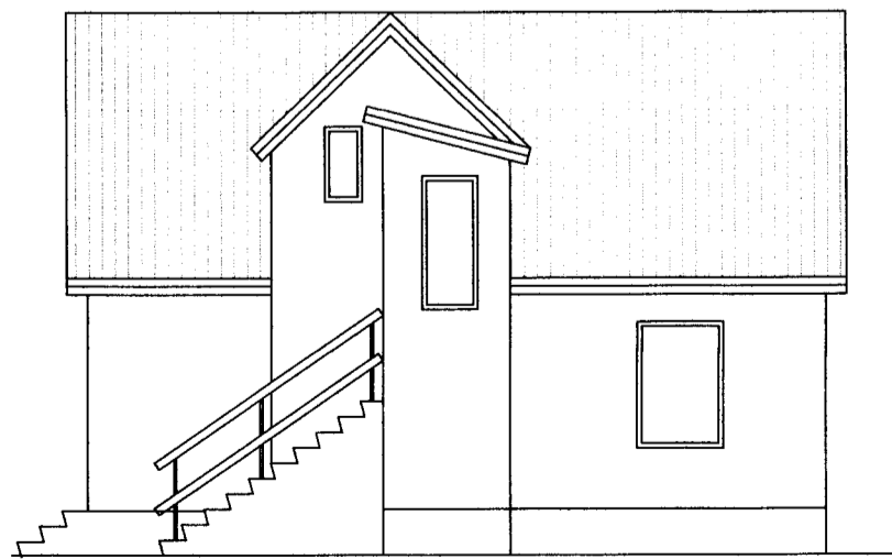
SUÐURHLIÐ 1:100
