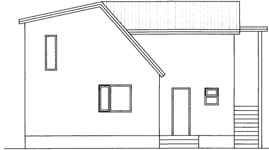
VESTURHLIÐ 1:100
