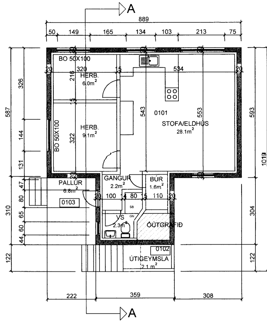
GRUNNMYND 1 HÆÐ 1:100
