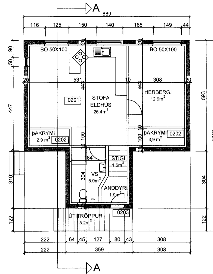
GRUNNMYND 2 HÆÐ 1:100
