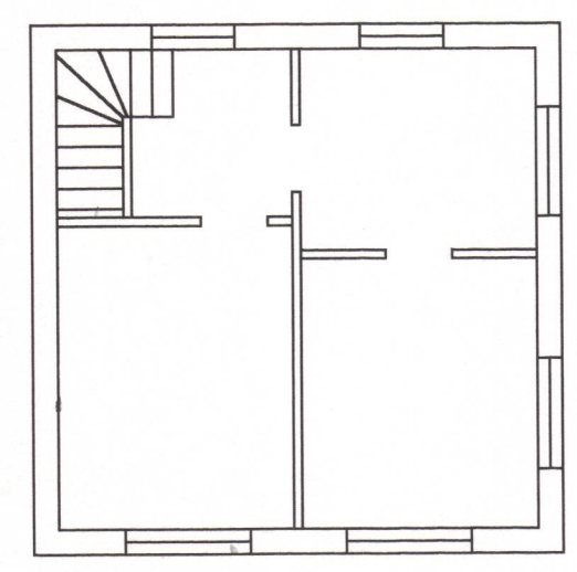
Grunnmynd efri hæð
